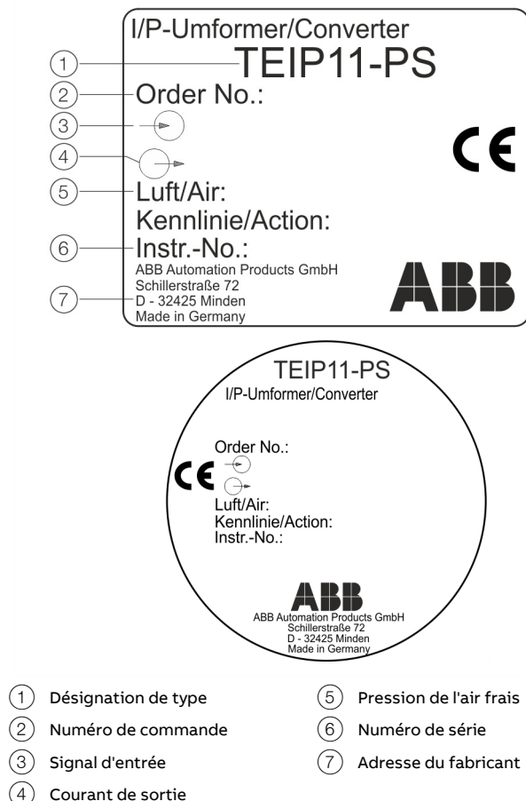
Figure 3 : Plaque signalétique (exemple)
