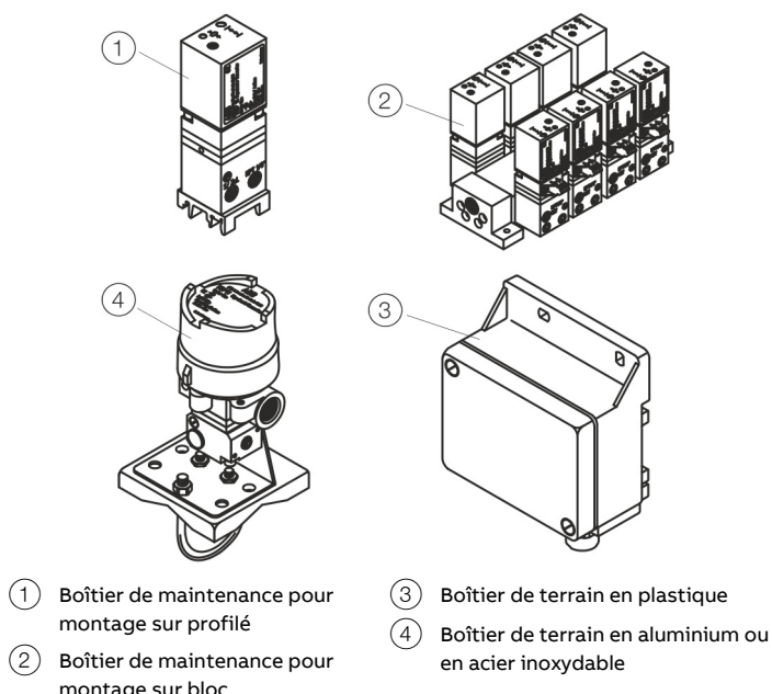
Figure 2 : Formes de construction TEIP11-PS
