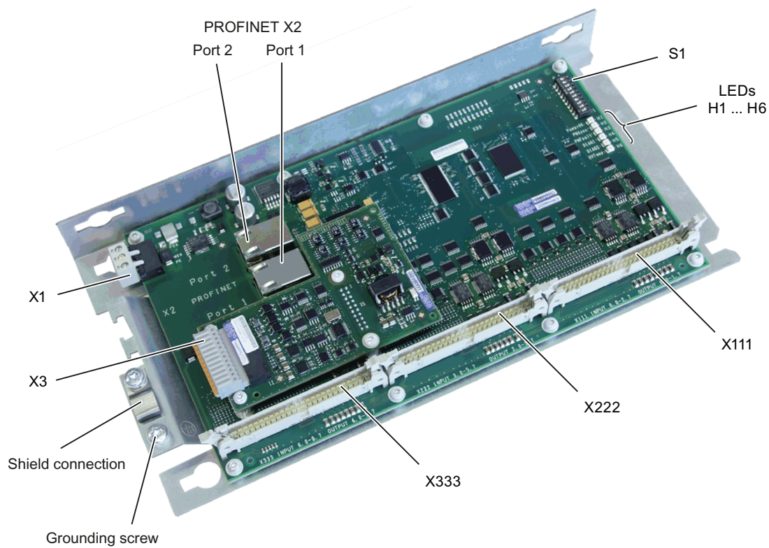
Figure 9-13 PP 72/48D 2/2A PN I/O module
