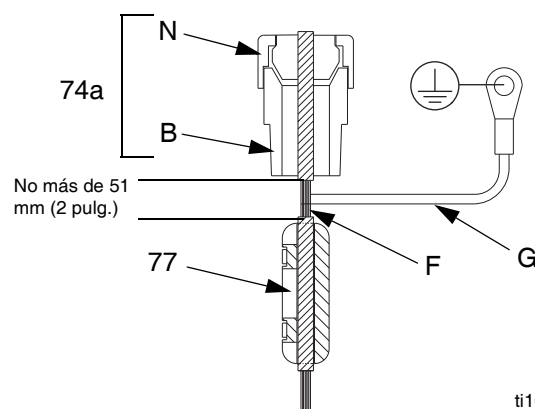
FIG. 13. Circuito del cable de campo de IS
