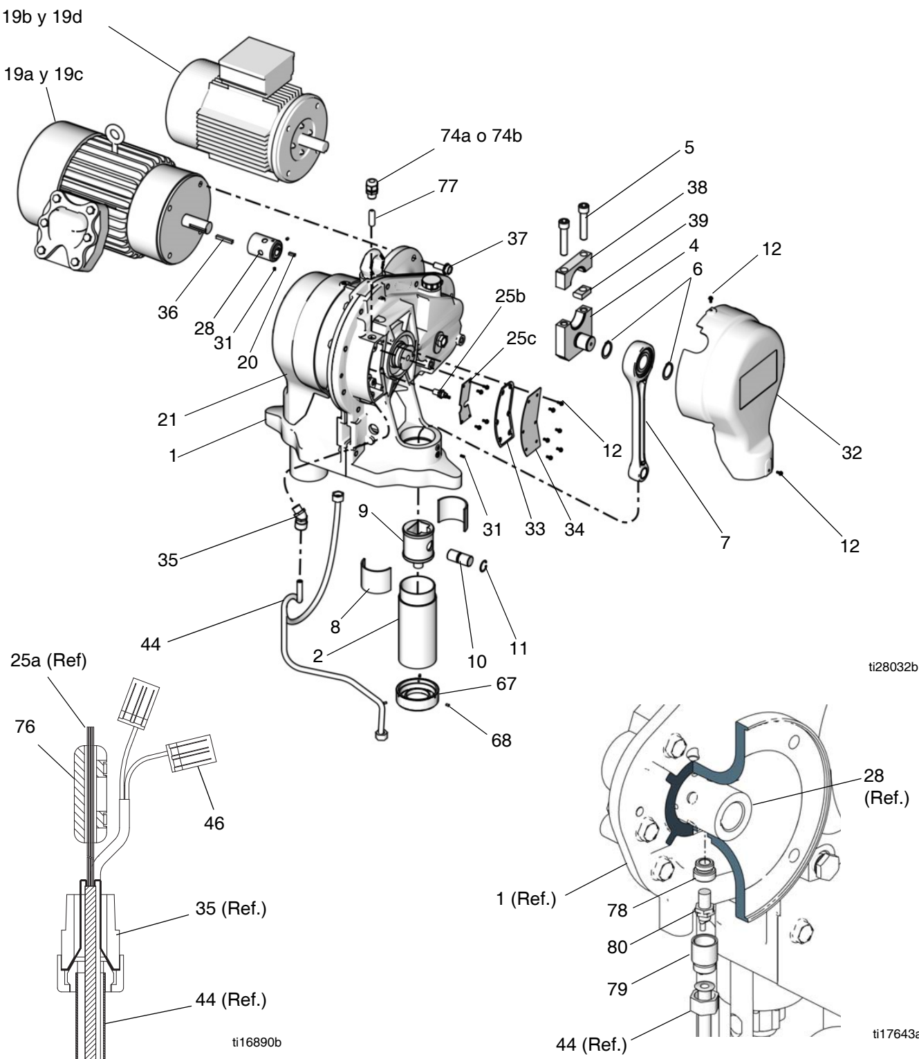
Piezas y ubicación de las piezas del sensor de posición
