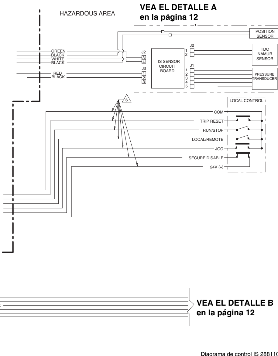
FIG. 2: Diagrama de cableado del sistema, para ubicaciones peligrosas
