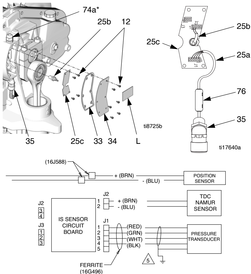
Diagrama de conexión a tierra del transductor de presión
