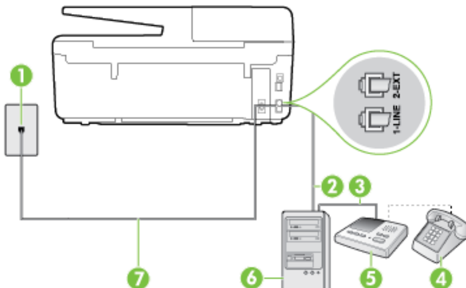
Figura B-13 Vista posterior de la impresora
