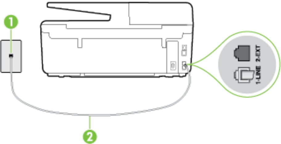
Figura B-3 Vista posterior de la impresora
