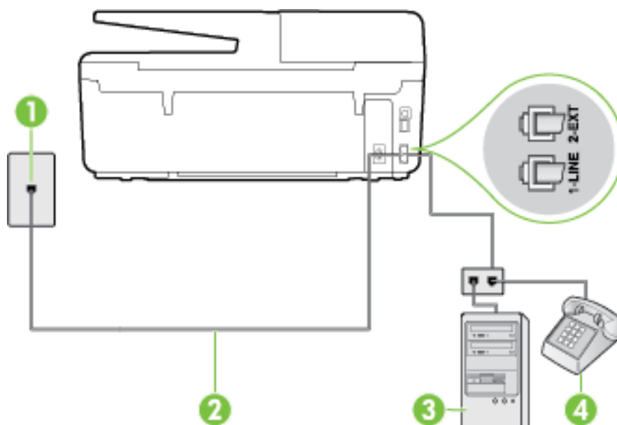
Figura B-16 Vista posterior de la impresora
