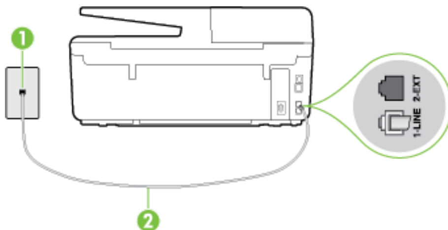
Figura B-1 Vista posterior de la impresora
