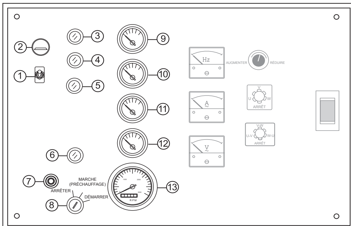
Figure 5. Panneau de commande du moteur
