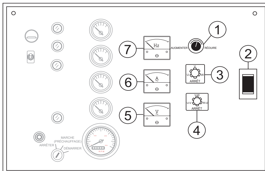
Figure 4. Panneau de commande du générateur
