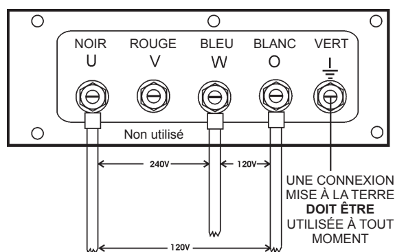
Figure 27. Cosses de sortie UVWO Connexions 1Ø-200/100V
