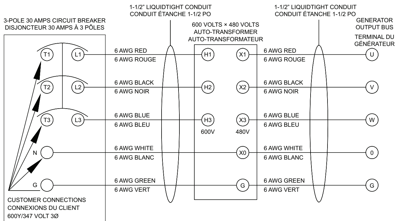
Figure 67. Schéma de câblage du transformateur automatique 600 V.c.a
