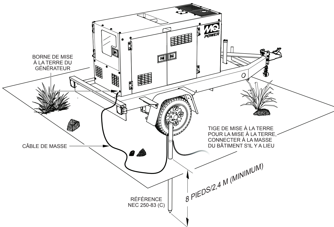
Figure 2. Application de mise à la terre typique du générateur
