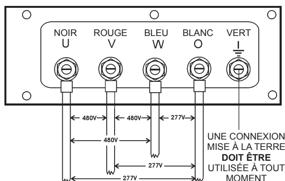
Figure 25. Cosses de sortie UVWO Connexions 3Ø-440/254V
