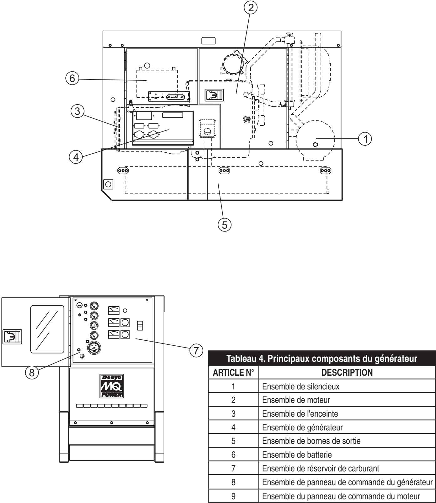
Figure 3. Composants principaux
