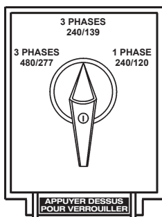
Figure 14. Commutateur de sélection de tension Position 3Ø 240/139V
