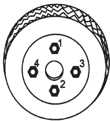
4 ÉCROUS DE ROUE
