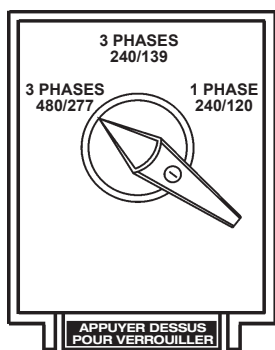
Figure 28. Commutateur de sélection de tension Position 3Ø-240/139V (transformateur automatique 600 V.c.a)
