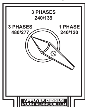
Figure 24. Commutateur de sélection de tension Position 3Ø-480/277V
