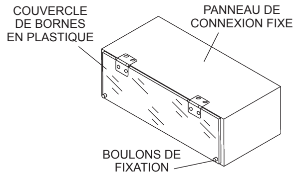
Figure 10. Couvercle en plastique (Cosses de sortie)
