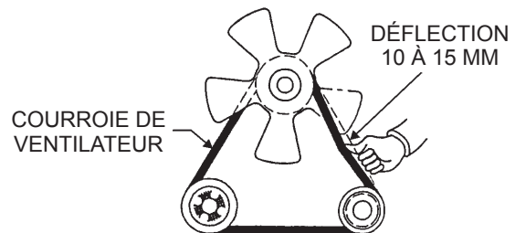
Figure 37. Tension de la courroie de ventilateur
