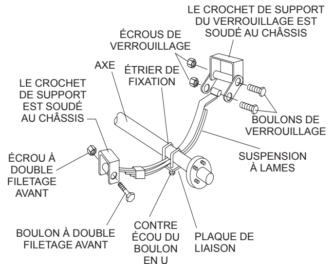
Figure 63. Composants de la suspension à lames
