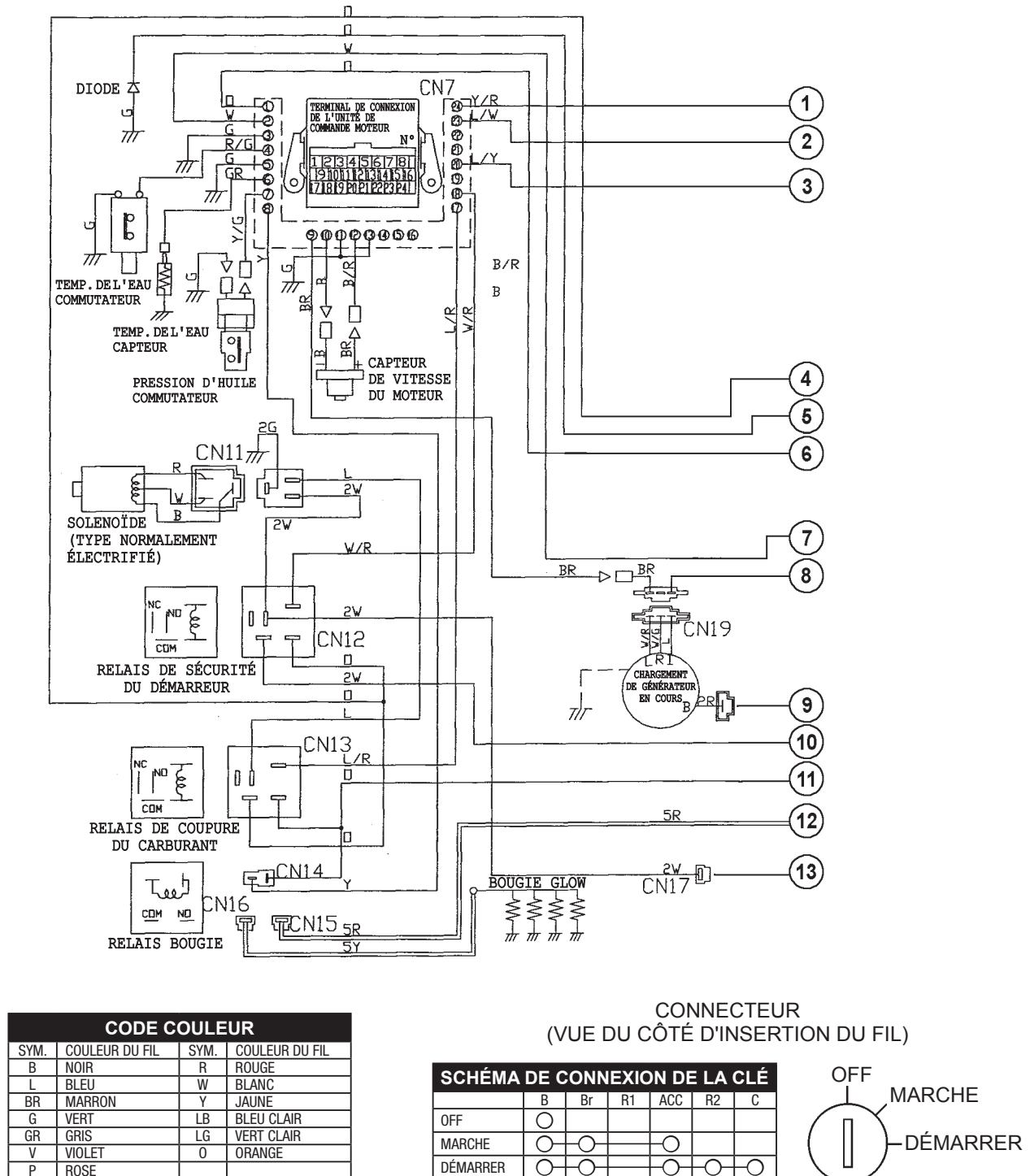
Figure 68. Schéma de câblage du moteur
