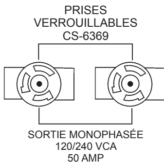
Figure 8. Prises auxiliaires verrouillables 120/240V
