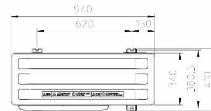
室外機 (CU-L140HA2 / CU-L140HA3)
