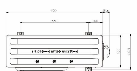
室外機 (CU-N140HA2 / CU-N140HA3)
