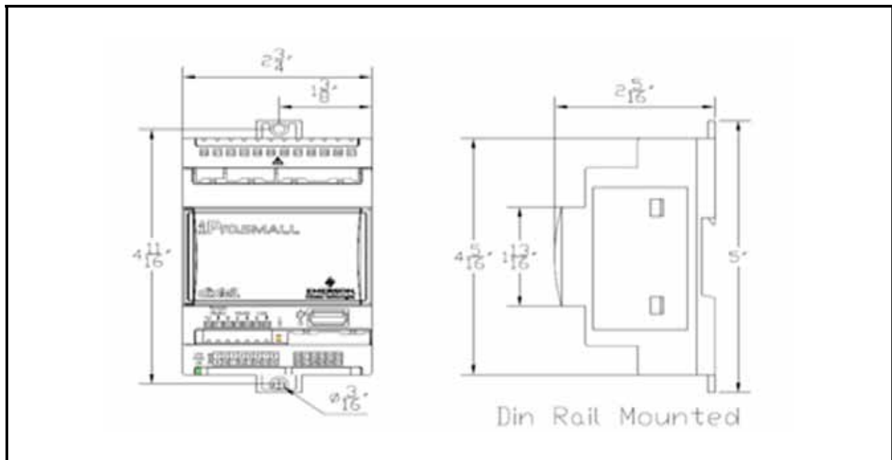
Figure 2-1 - DIN Mounting
