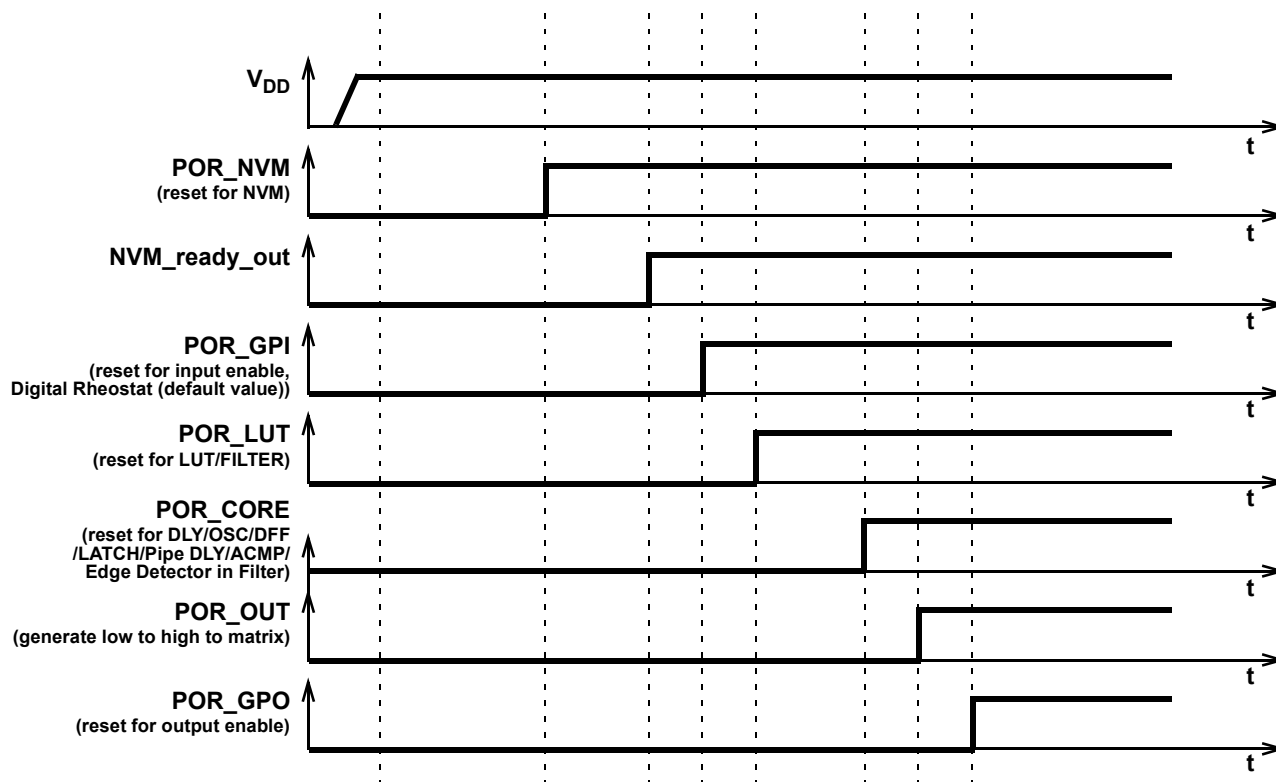
Figure 223: POR Sequence
