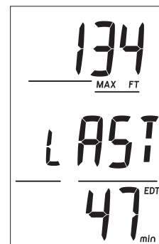
Fig. 4 - NORM SURF ALT 1 (Last dive's data)
