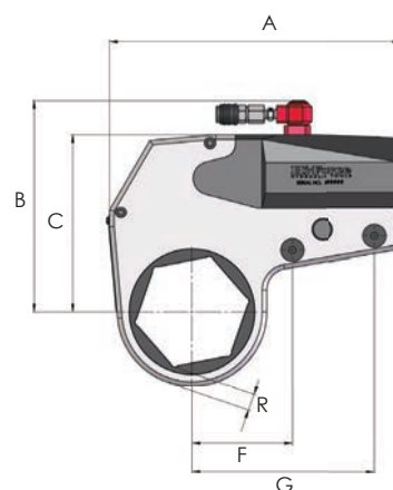
TWH430N (cuerpo de acero)
