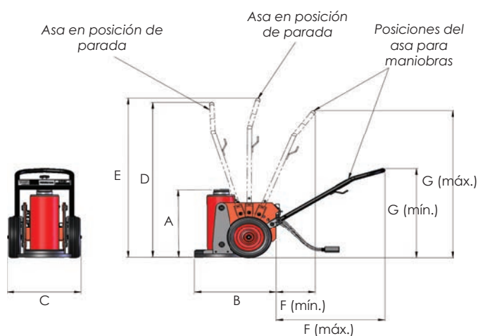
Dimensiones para todos los demás modelos:
