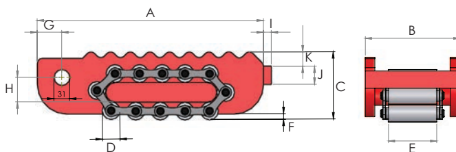
Planos de los modelos RSN60 y RSN80
