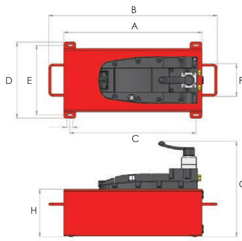
AHP1141 (depósito de aceite hecho de metal) AHP1142 (depósito de aceite hecho de metal)
