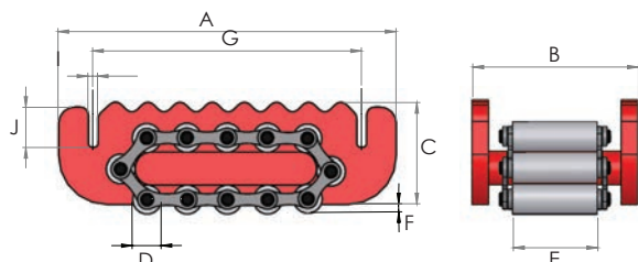
Planos de los modelos RSN10, RSN15 y RSN30
