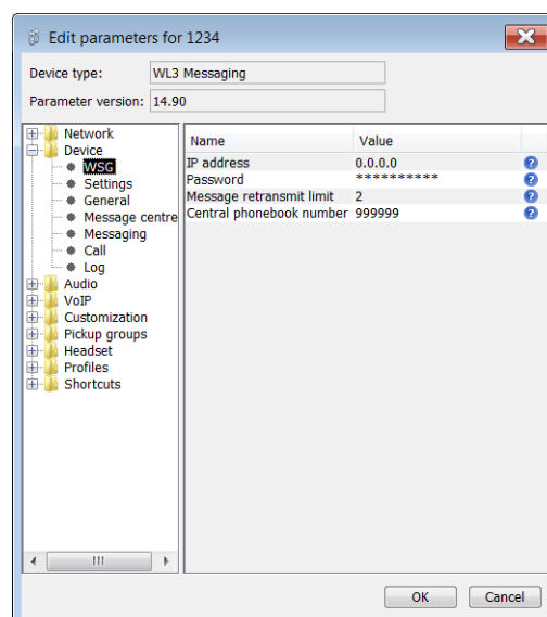
Figure 15. Editing parameters
