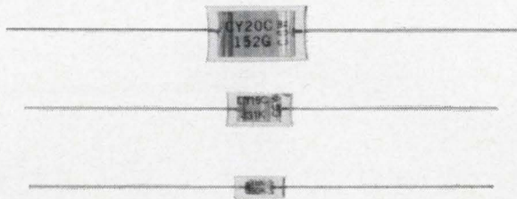
CORNING CYFM Capacitors: CYFM 10, 0.5—300 pf; CYFM 15, 220—1200 pf; CYFM 20, 560—5100 pf; CYFM 30, 3600—10,000 pf; VDCW, 300 and 500 volts.
