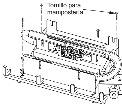
Figura 13 - Instalación de la base en el suelo de la chimenea
