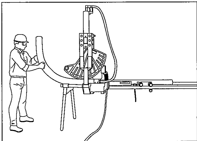
53. Retire el tubo portacables de la dobladora.
