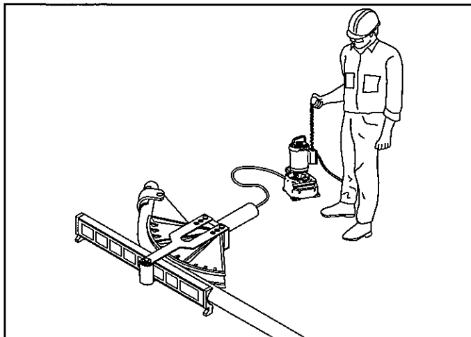
15. Cintre de 45°.
