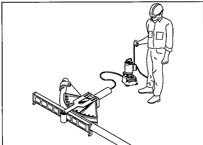
15. 45° de doblez.
