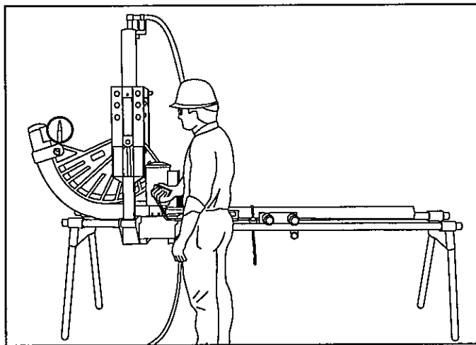
45. 60° de doblé.
