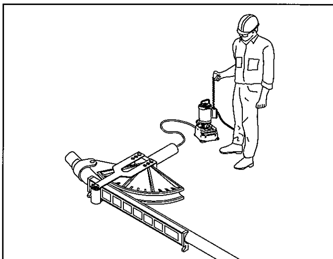
14. Cintre de 10°.
