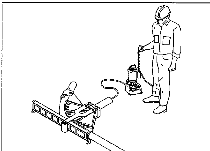
16. Cintre de 60°.
