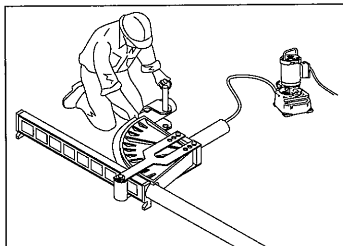
19. Retire la clavija de la silla.
