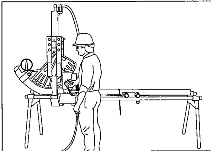
44. 45° de doblé.
