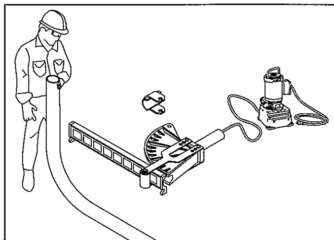
20. Le cintrage de 90° est terminé.
