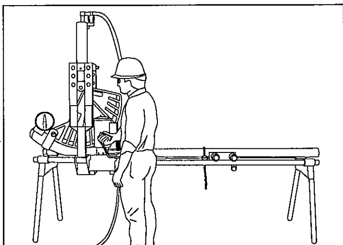
42. 15° de doblé.
