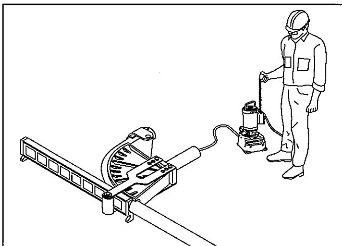
17. Cintre de 90°.
