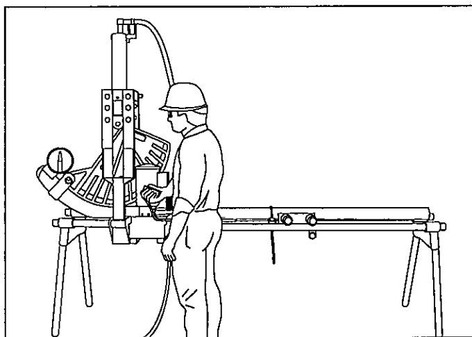
43. 30° de doblé.
