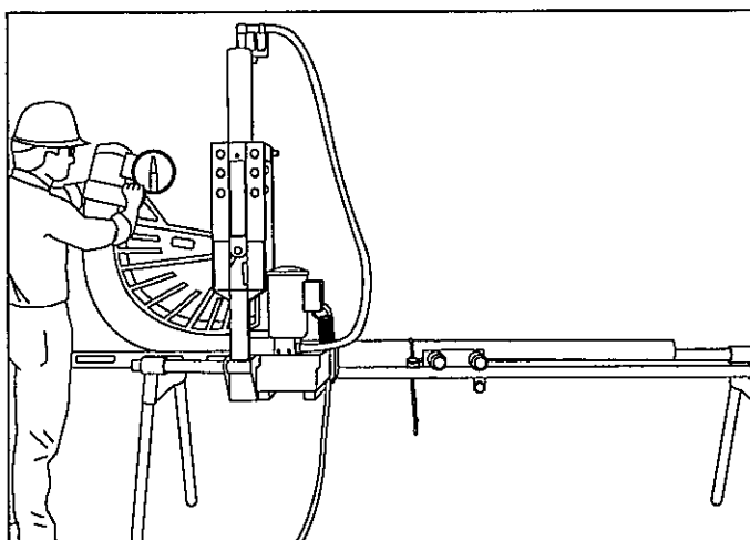
48. Quite el indicador de grados de dobléz 1805.
