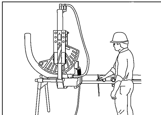
52. Desserrer la chaîne de l'étau.
