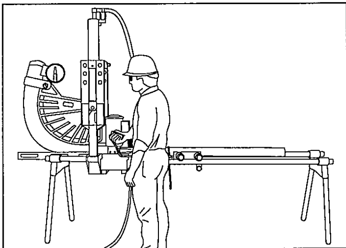
47. 90° de dobléz.
