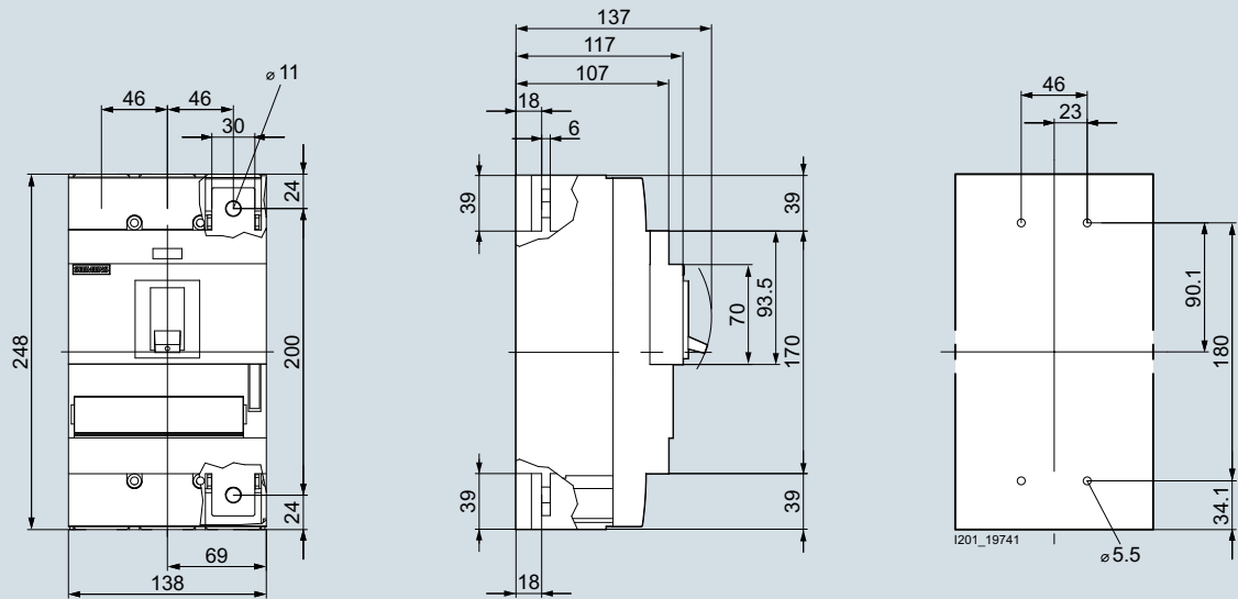
3VM13/14, 3 polos
