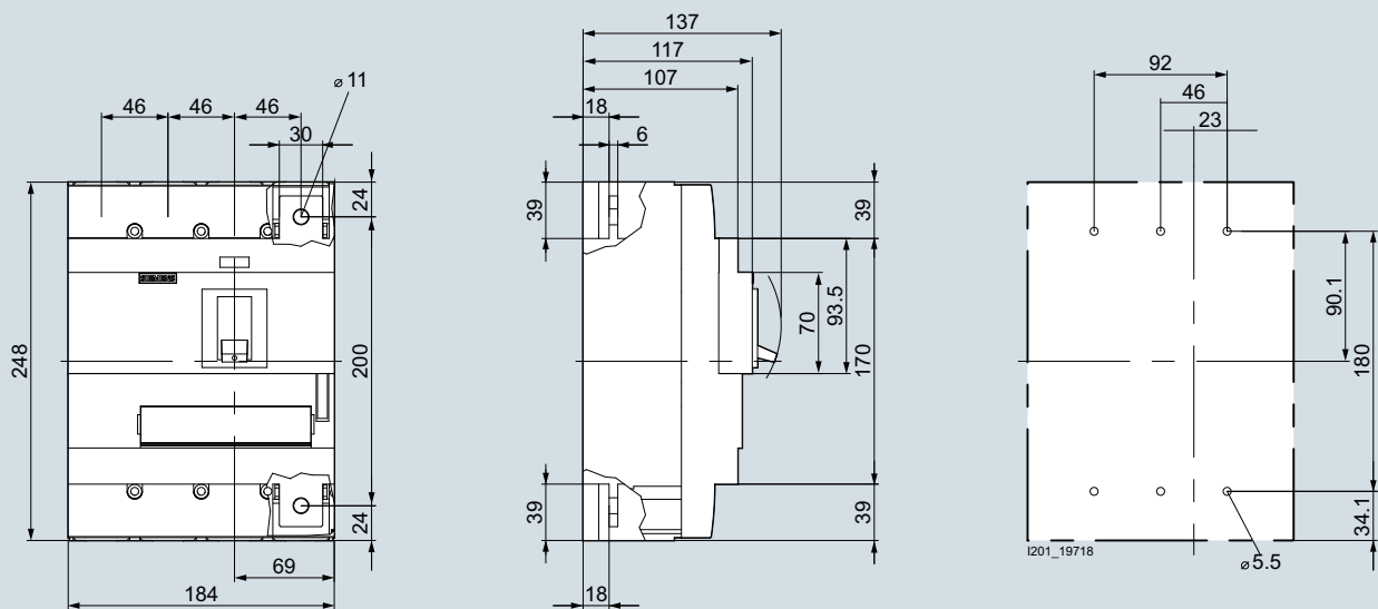
3VM13/14, 3 polos
