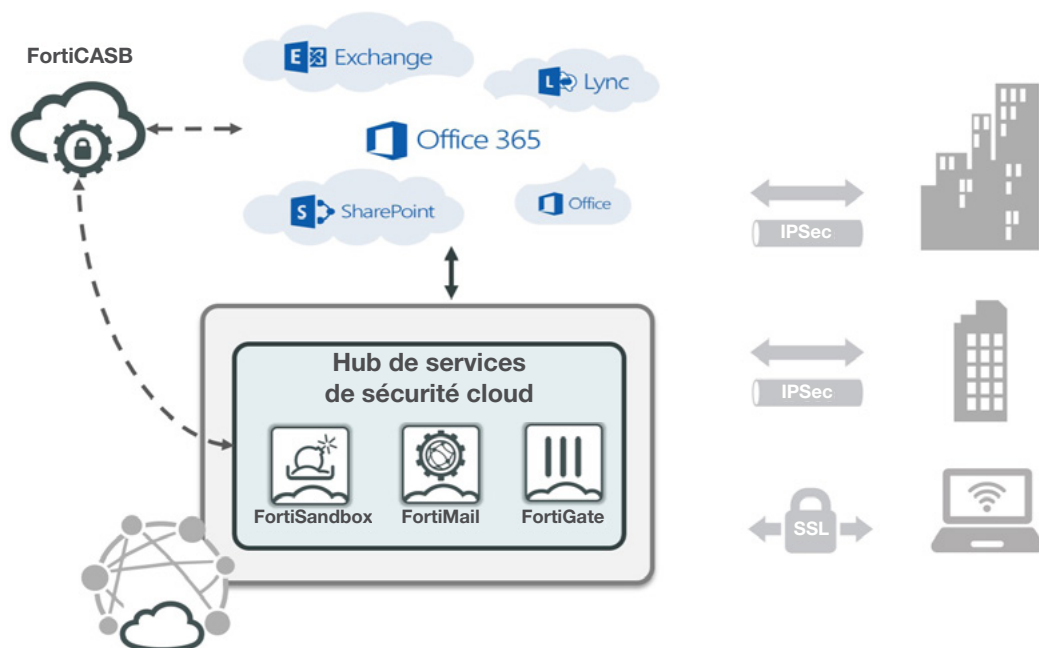
Schéma 12. Une productivité sécurisée dans le cloud par Fortinet.
