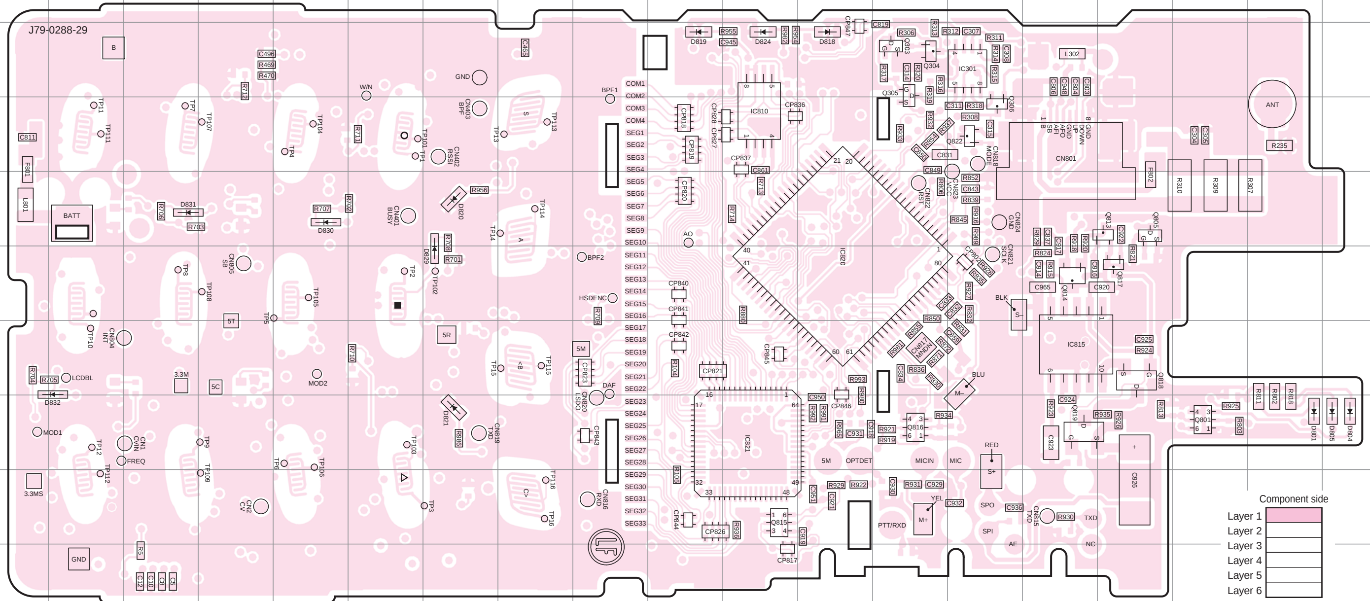
TX-RX UNIT (X57-7890-71) Component side view (J79-0288-29)
