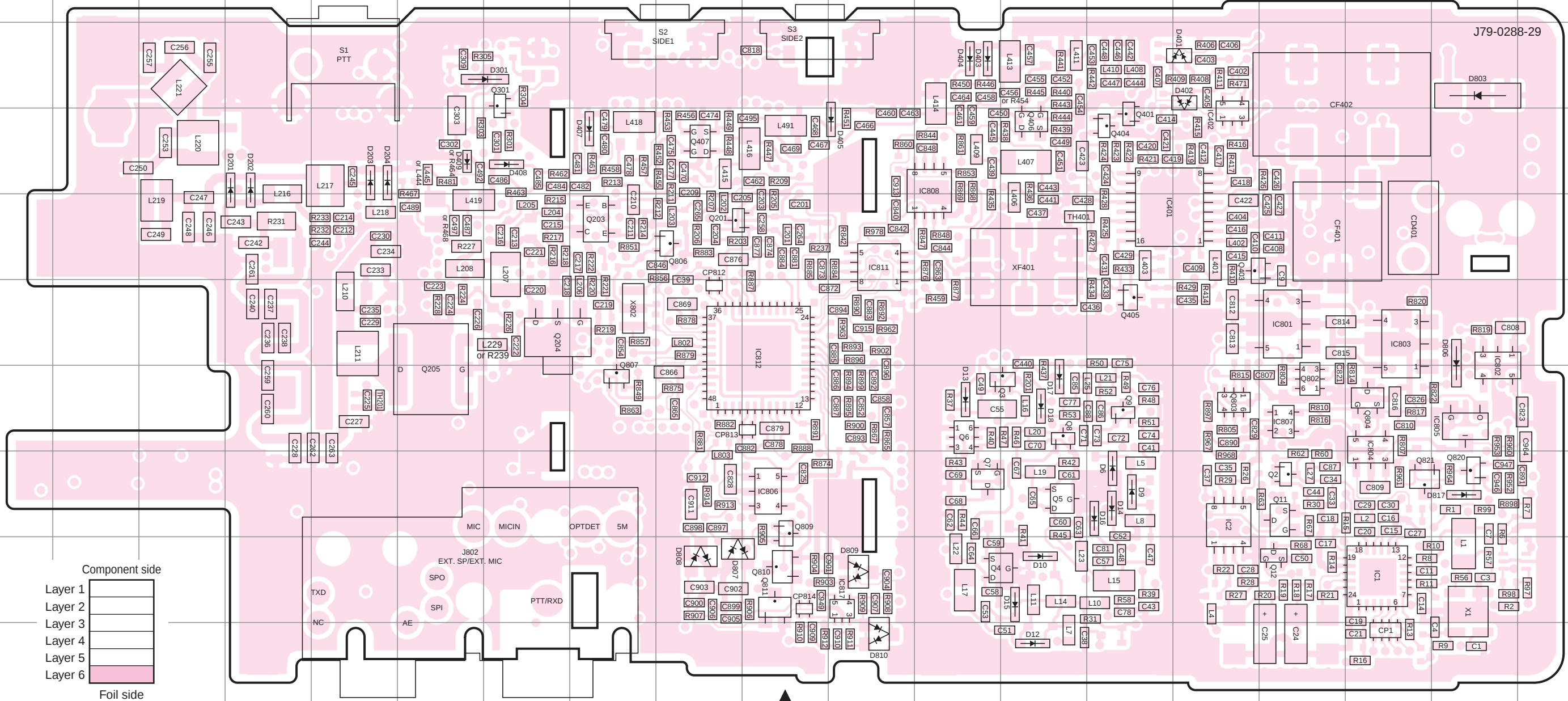
TX-RX UNIT (X57-7890-71) Foil side view (J79-0288-29)
