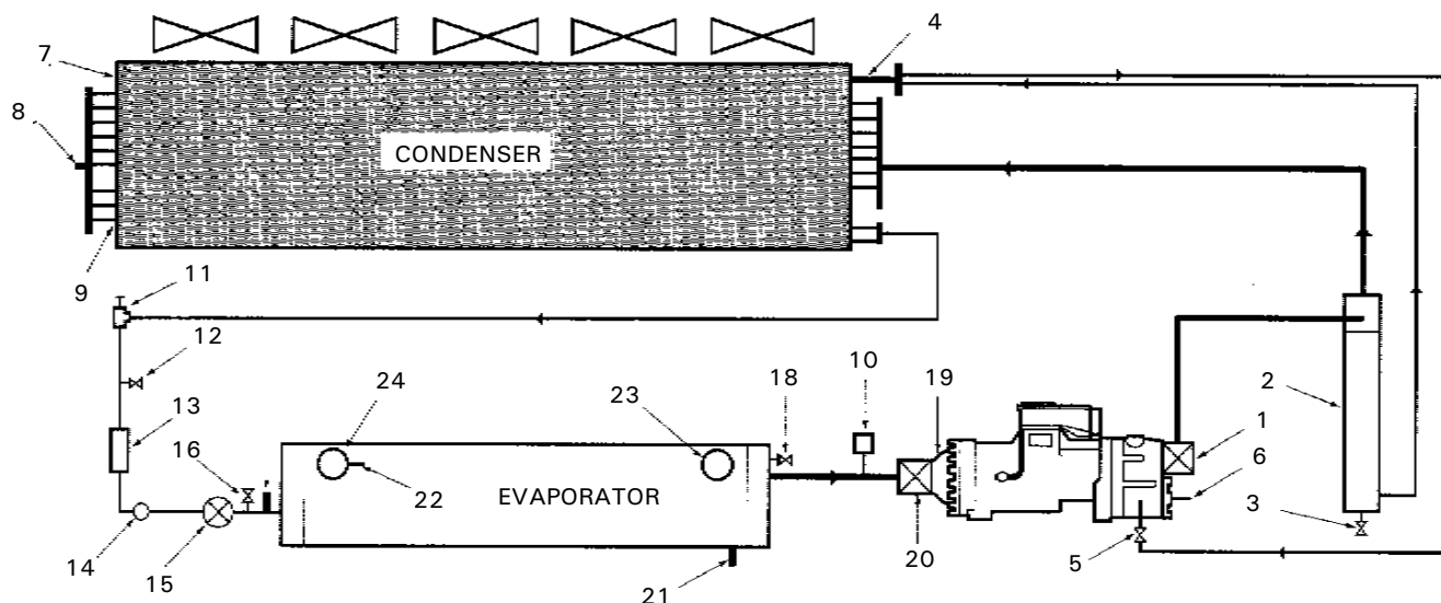
Figura 21: Sistema de refrigeração e componentes de unidade RTAA
