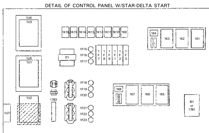
Figura 25: Painel de controle das unidades RTWA.
