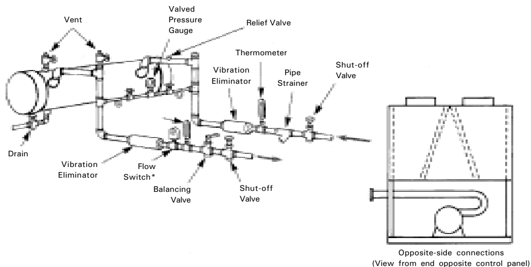
Figura 8: Componentes da tubulação de água do evaporador
