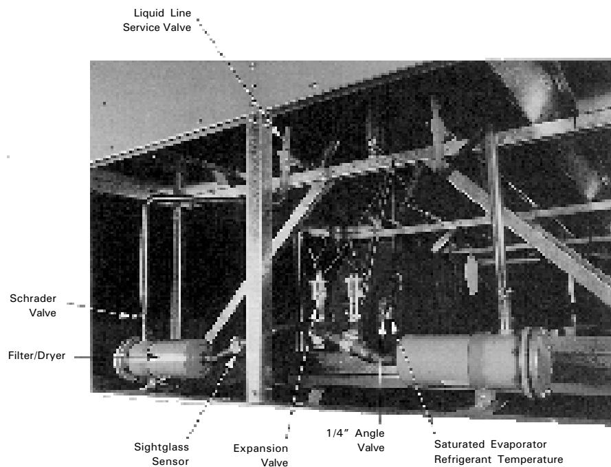
Figura 2: Típico resfriador de líquido RTAA 70-125 TRs — Vista posterior / Lado externo
