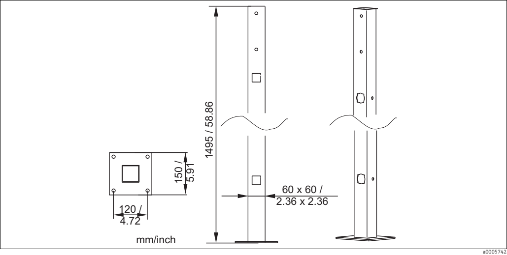
Fig. 34: Universal post
