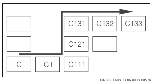
Fig. 20: Function coding
