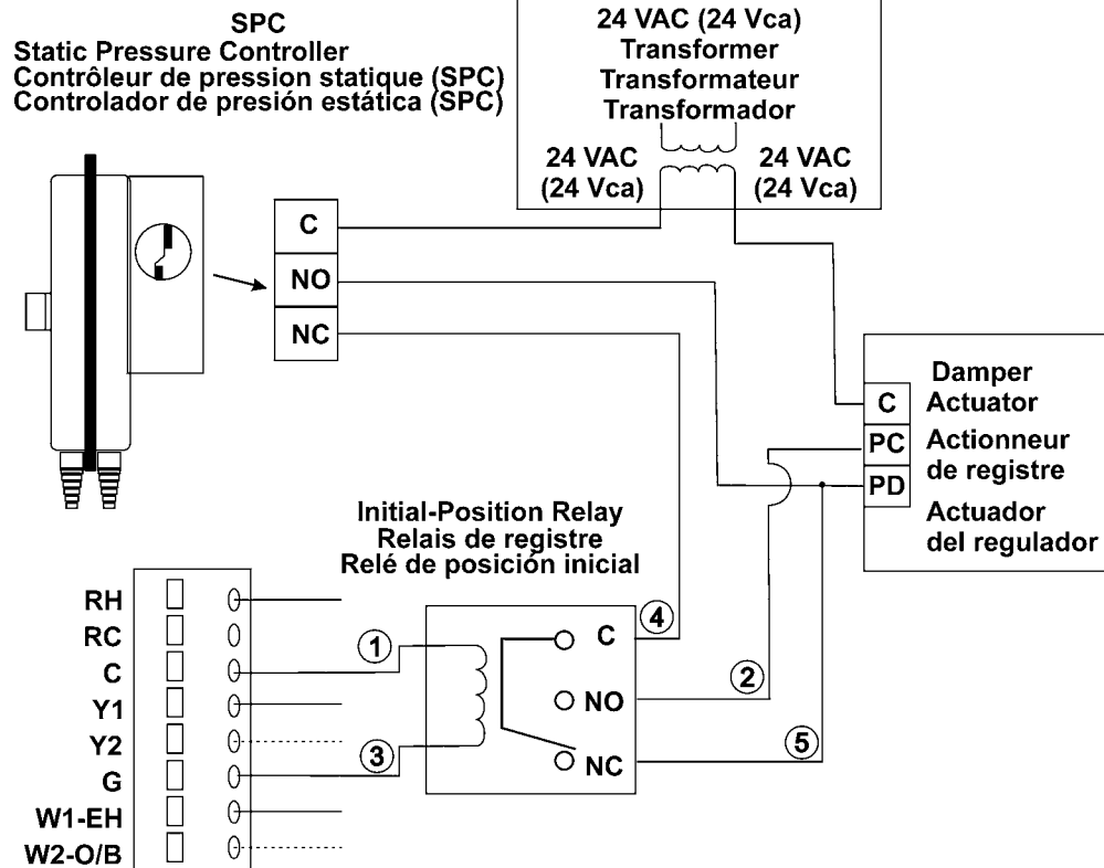
Figure 2 – Schéma de câblage
