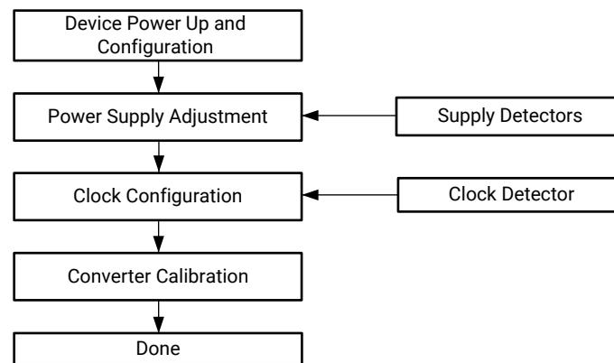
Figure 78: POR Finite State Machine
