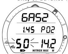
Fig. 23 - Set FO2 GAS 2 (50% O2)
