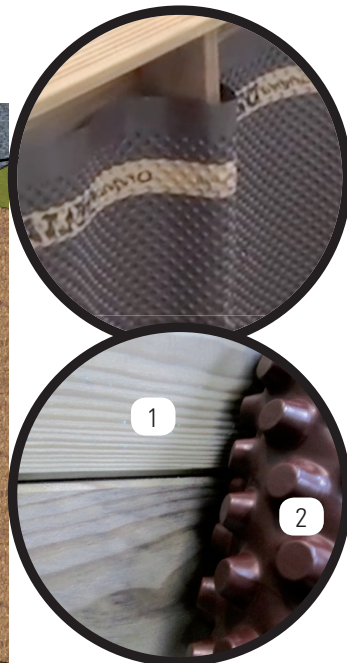
1- Composite frame 2- Rol HDPE-noppenfolie ter bescherming en voor de drainage
