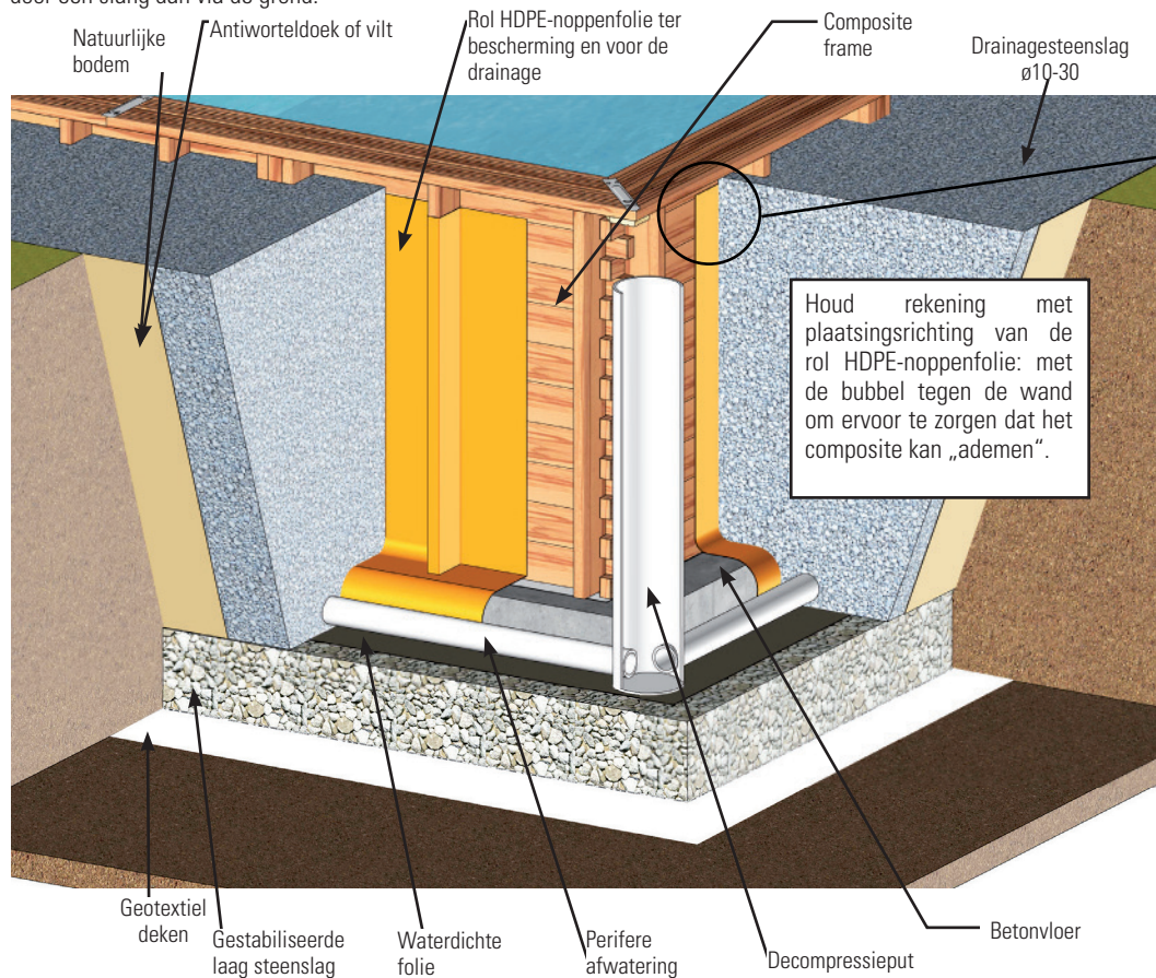
1- Composite frame 2- Rol HDPE-noppenfolie ter bescherming en voor de drainage
