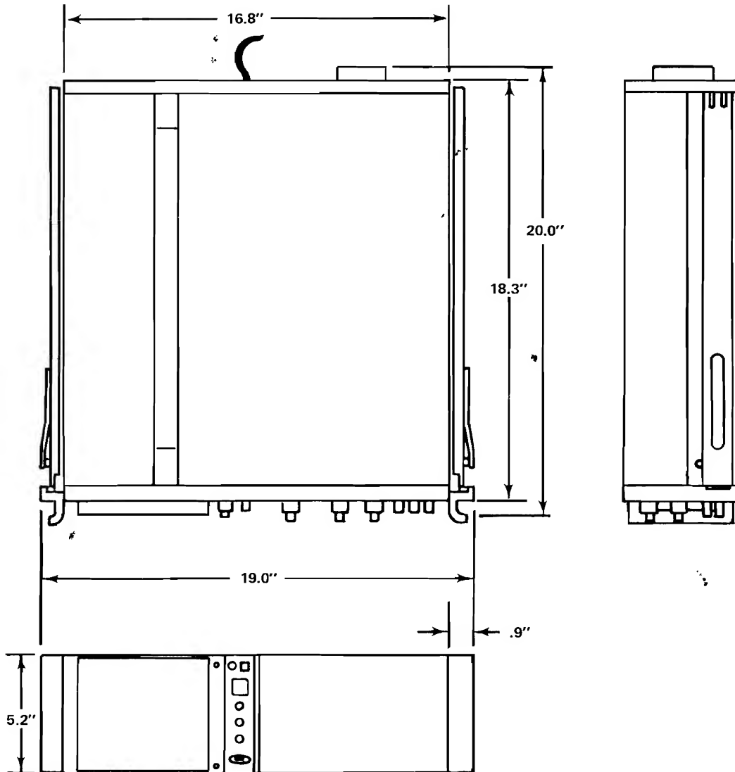
Fig. 6-2. Dimensional diagram.
