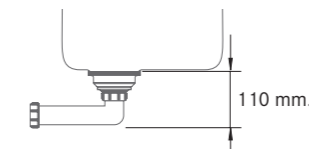
Distancia ocupada por debajo del fregadero Válvulas (A, B, BG, C, D y DG) + codo del Sifón (SF1, SF2)
