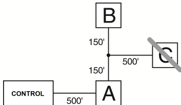
Figura 1-1 Cableado Corbus
