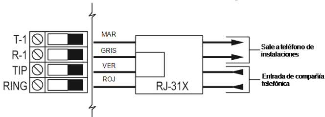
Figura 1-6 Cableado de línea telefónica
