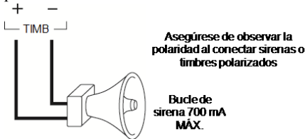
Figura 1-5 Cableado de terminales sirena
