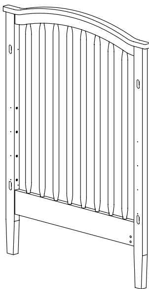
B. RIGHT CRIB END
