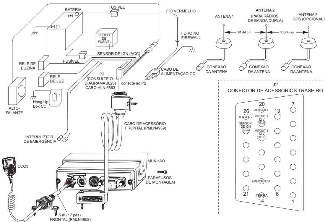
Figura 2-9. Instalação do Rádio (O3, Potência Média, Montagem Remota)
