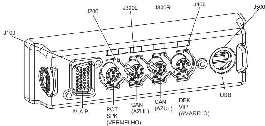
Figura 2-18. Diagramas da Cabeça de Controle Remota
