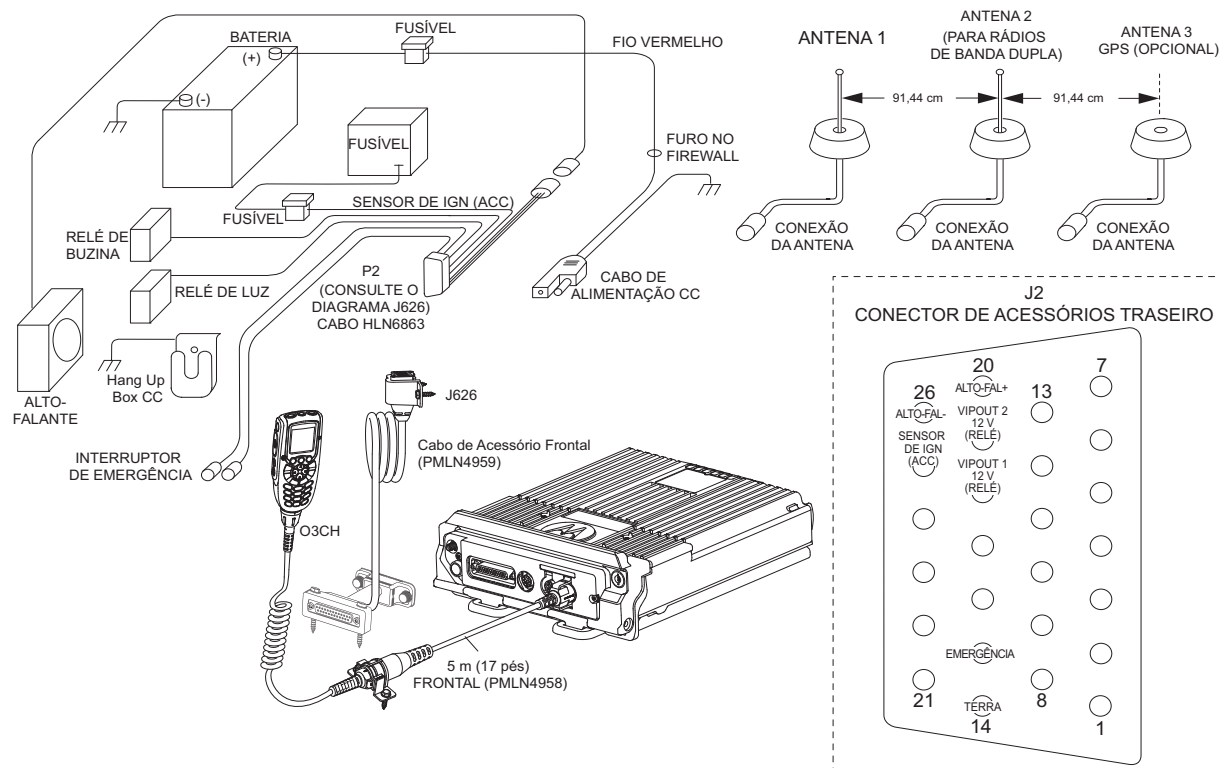
Figura 2-13. Instalação do Rádio (O3, Potência Alta, Montagem Remota)
