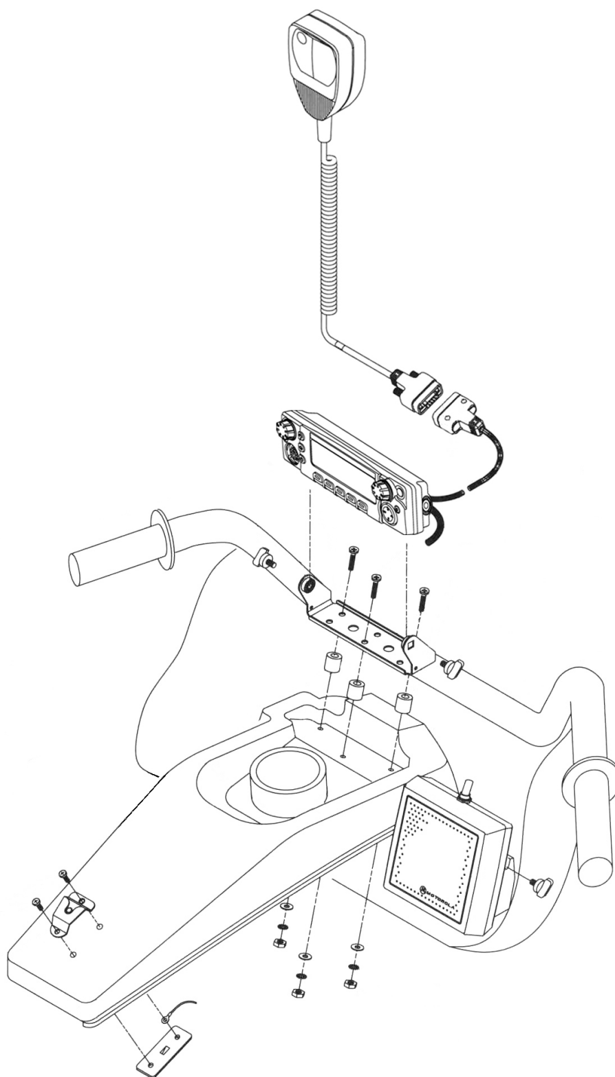
Figura 5-7. Instalação no Console do Tanque de Combustível com Alto-falante e Cabeça de Controle Montados Separadamente
