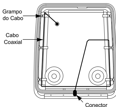
Figura 5-11. Roteamento do Cabo Coaxial do GPS
