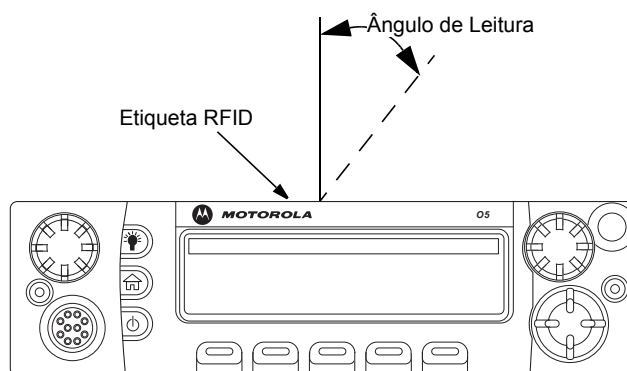
Figura 2-64. Ângulo de Leitura do Rádio de Potência Média
