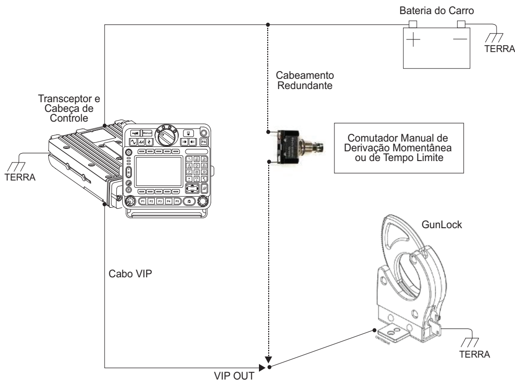
Figura 4-4. Diagrama da Redundância do Interruptor de Gunlock
