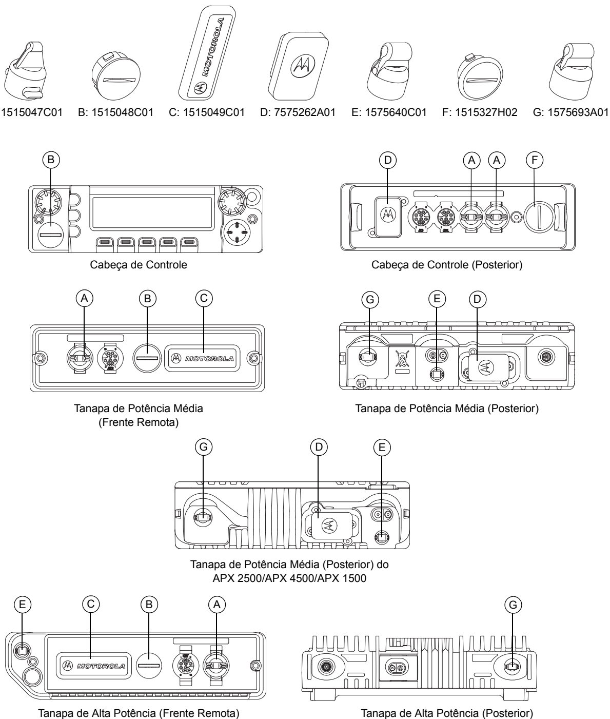
Figura 6-1. Locais de Instalação das Tampas de Poeira
