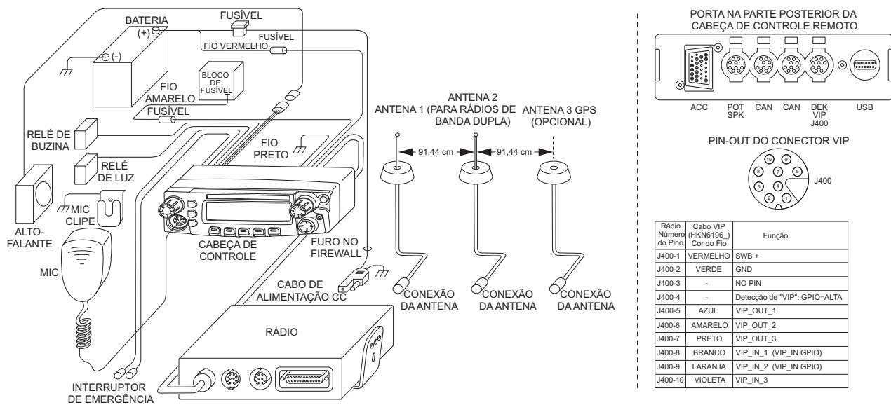
Figura 2-10. Instalação do Rádio (O5, Potência Média, Montagem Remota)
