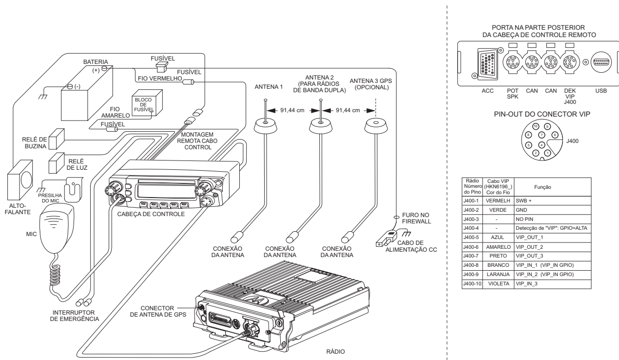
Figura 2-14. Instalação do Rádio (O5, Potência Alta, Montagem Remota)
