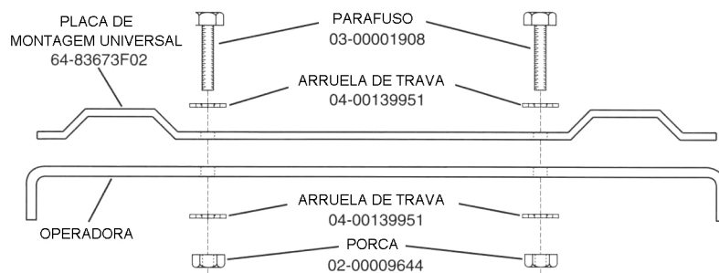
Figura 5-2. Instalação da Placa de Montagem Universal (Peça do Kit de Compartimento de Rádio)
