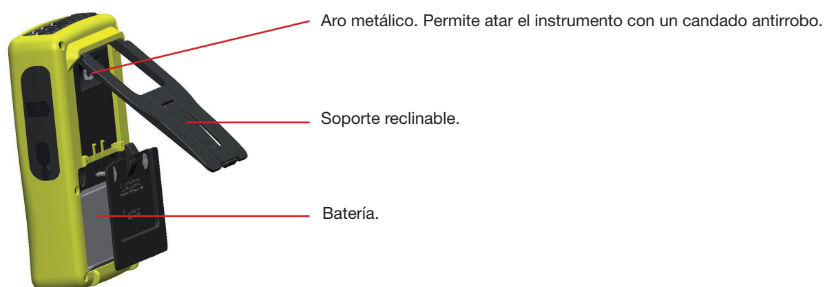
Figura 5: soporte y tapa de acceso a la batería
