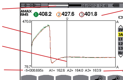
Figura 44: la pantalla de visualización RMS en 3A para una conexión trifásica con neutro
