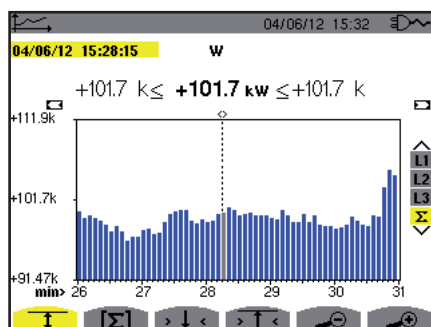
Figura 100 W ( \Sigma ) con MIN-AVG-MAX
