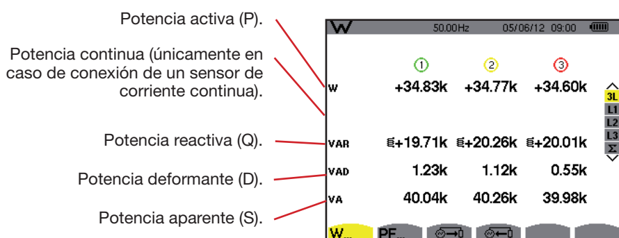
Figura 109: la pantalla de las potencias en 3L
