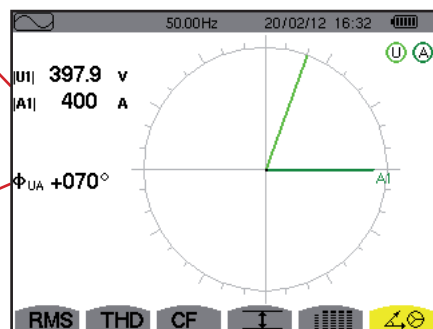
Figura 84: la pantalla de visualización del diagrama de Fresnel en Bifásico de 2 hilos
