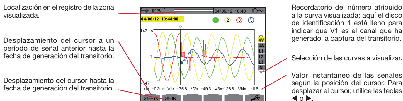
Figura 41: ejemplo de visualización de los transitorios en forma de curvas con conexión trifásica de 5 hilos
