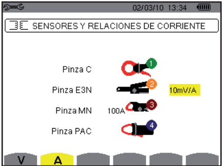
Figura 25: la pantalla Sensores y ratios de corriente en el menú Sensores y ratios
