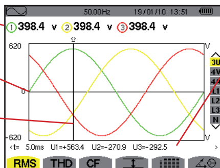
Figura 63: la pantalla de visualización RMS en 3U
