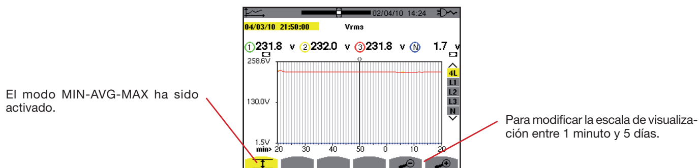
Figura 92: Vrms (4L) con MIN-AVG-MAX
