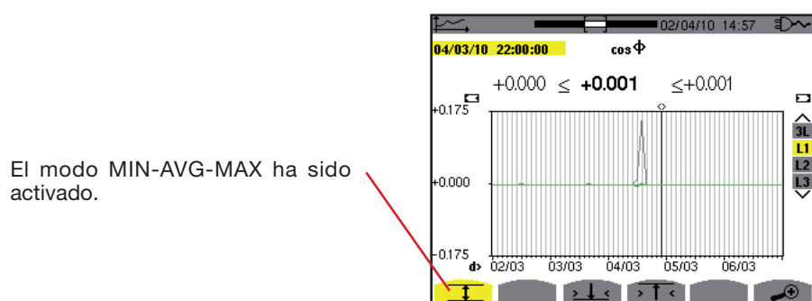
Figura 104: cos \Phi (L1) con MIN-AVG-MAX
