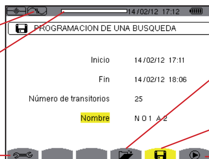
Figura 38: la pantalla Programación de una búsqueda en modo transitorios
