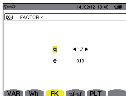
Figura 22: el menú Selección de los coeficientes de cálculo del factor
