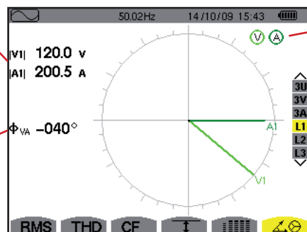
Figura 83: la pantalla de visualización del diagrama de Fresnel en L1
