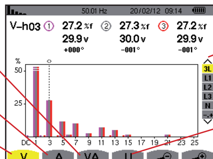
Figura 51: la pantalla del modo armónico
