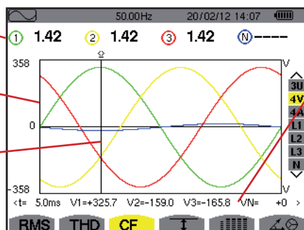
Figura 71: la pantalla de visualización CF en 4V
