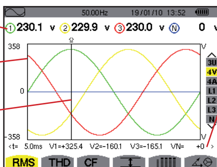
Figura 64: la pantalla de visualización RMS en 4V
