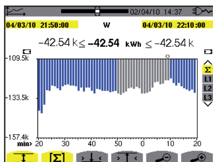
Figura 102: Wh ( \Sigma ) con MIN-AVG-MAX
