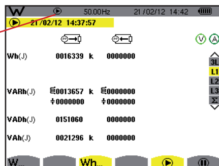
Figura 118: la pantalla de medición de energía en Julio
