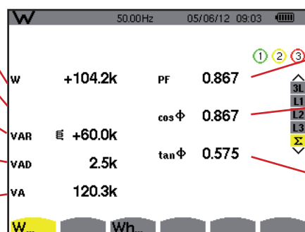
Figura 115: la pantalla de visualización de las potencias y magnitudes asociadas en \Sigma
