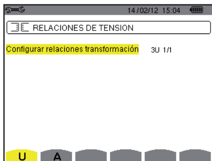
Figura 26: la pantalla Ratios de tensión en el menú Sensor y ratios en el caso de un montaje sin neutro
