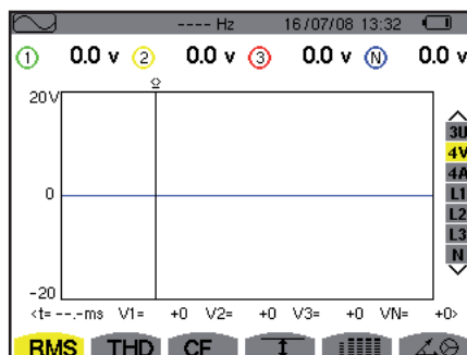
Figura 7: la pantalla Formas de onda
