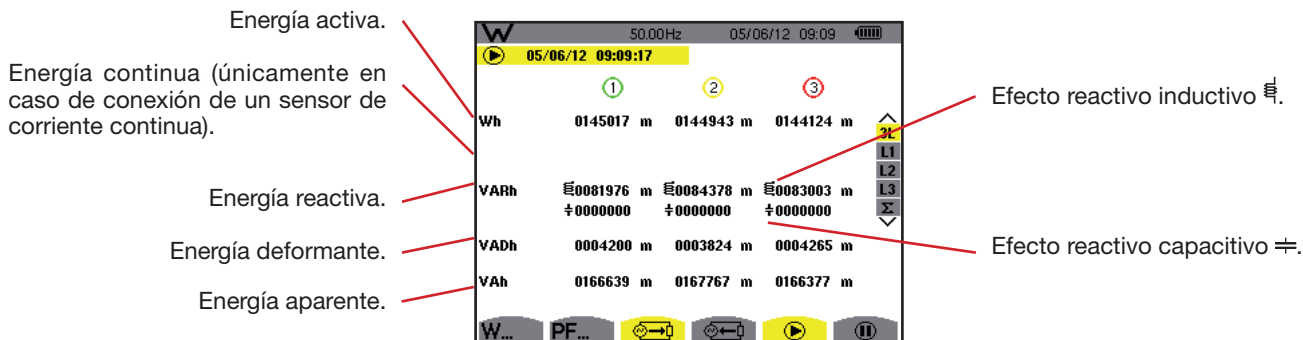
Figura 111: la pantalla de visualización de las energías consumidas en 3L
