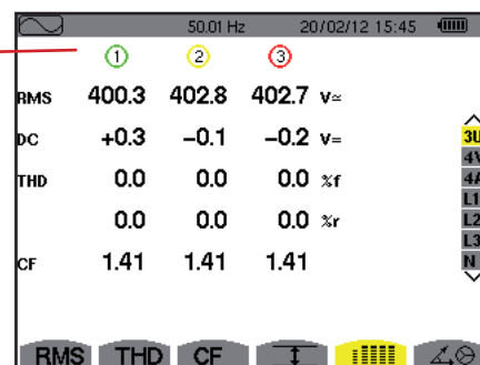
Figura 78: la pantalla de visualización simultánea en 3U
