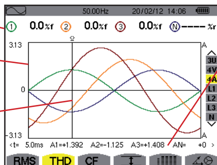
Figura 69: la pantalla de visualización THD en 4A
