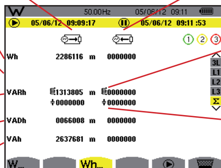
Figura 116: la pantalla de visualización de las sumas de las energías consumidas y aportadas en \Sigma
