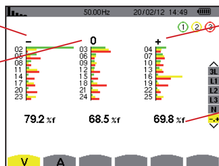
Figura 60: la pantalla del modo experto para la tensión de fase (montajes trifásicos con neutro)
