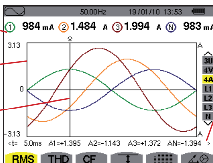
Figura 65: la pantalla de visualización RMS en 4A
