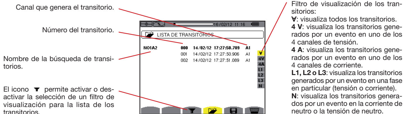
Figura 40: la pantalla Lista de los transitorios en el caso de un montaje trifásico de 5 hilos
