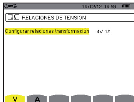
Figura 27: la pantalla Ratios de tensión en el menú Sensor y ratios en el caso de un montaje con neutro
