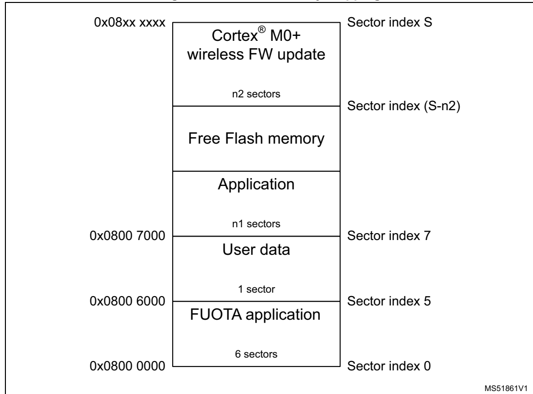
Figure 29. FUOTA memory mapping
