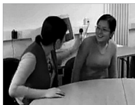
H.264
