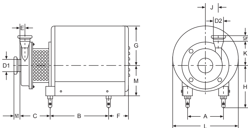
SFB-25外形安装尺寸 Dimensions
