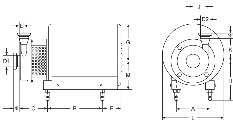
SFB-15外形安装尺寸 Dimensions
