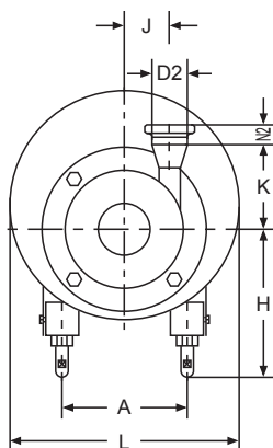
SFB-45外形安装尺寸 Dimensions
