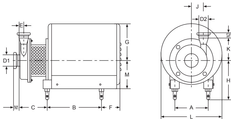
SFB-35外形安装尺寸 Dimensions
