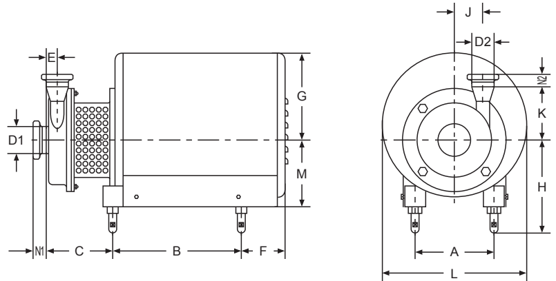
SFB-50外形安装尺寸 Dimensions
