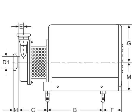
SFB-45外形安装尺寸 Dimensions
