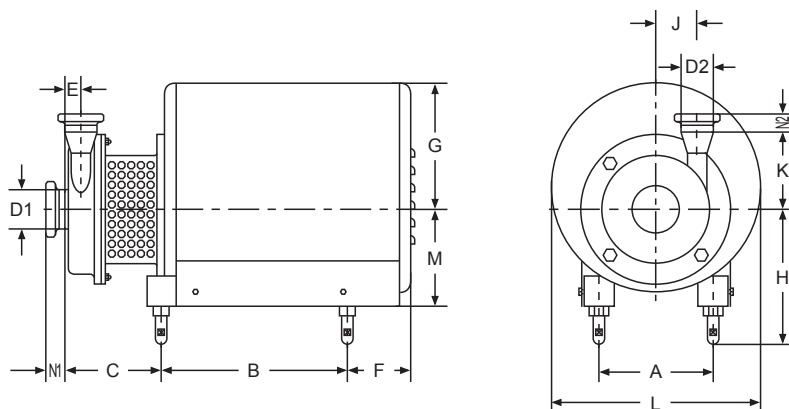
SFB-30外形安装尺寸 Dimensions
