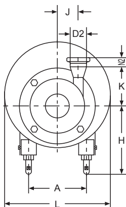
SFB-60外形安装尺寸 Dimensions
