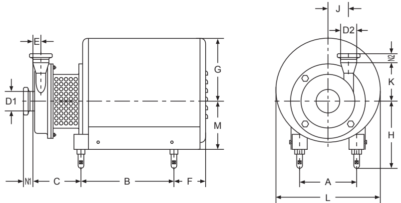
SFB-20外形安装尺寸 Dimensions
