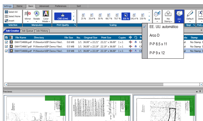
Control de carpeta de PC, navegador y controlador
