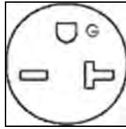
NEMA 6-20R Receptacle
