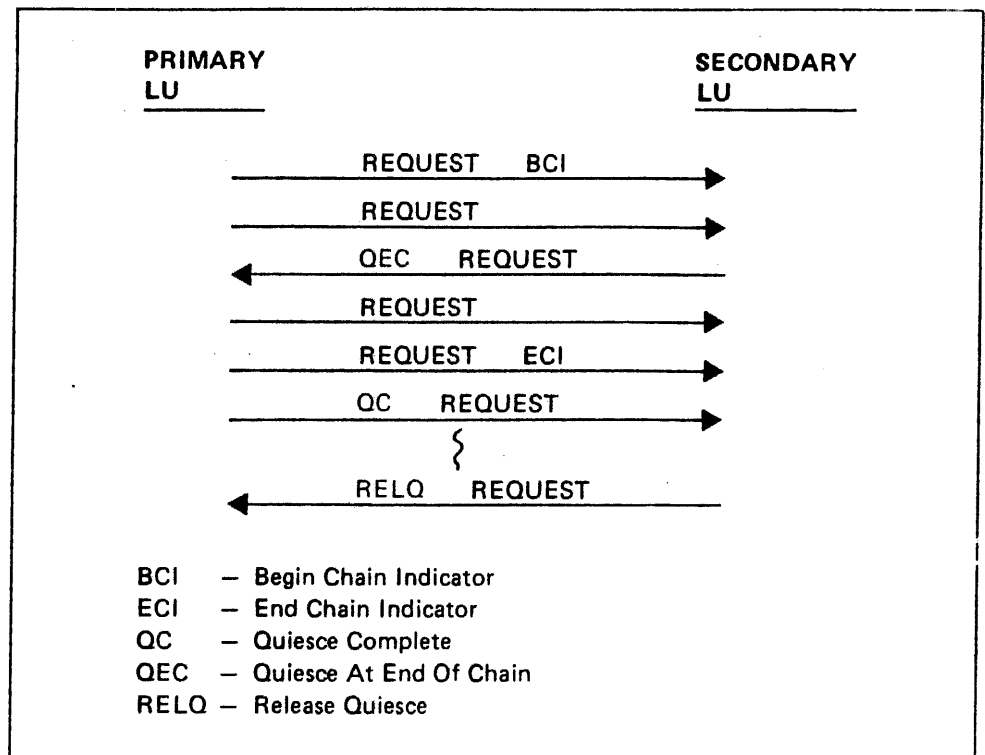
Figure 9-1. Quiesce Protocol
