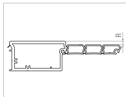
Fig. 4-18 Tambour door offset (O)
