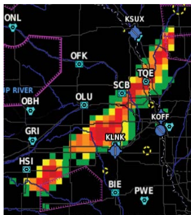
NEXRAD Data
