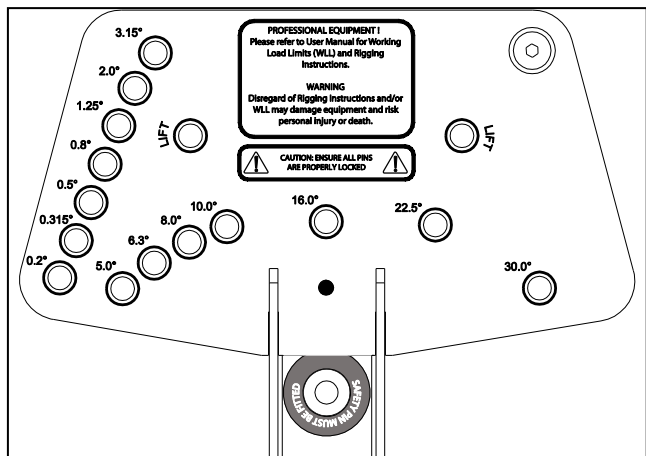
GEO S12 XBOW ANGLE SETTINGS PLATE
