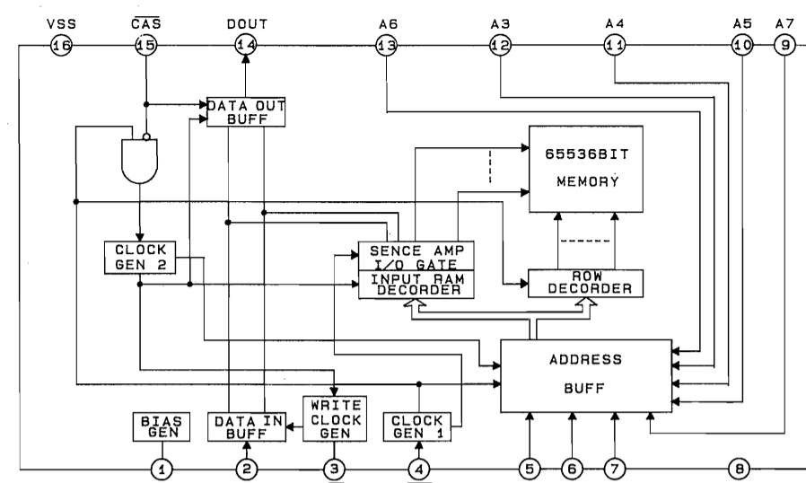
IC303 LM3364K-15
