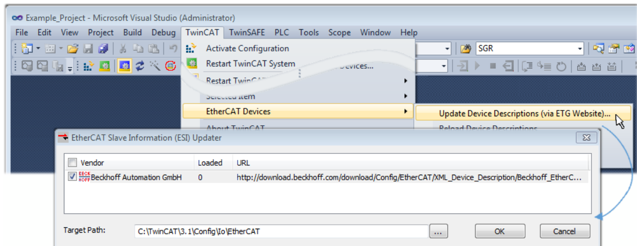
Fig. 102: Using the ESI Updater (TwinCAT 3)
