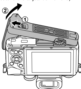
Desacoplamiento de la parte inferior de la empuñadura (para cambiar la batería o la tarjeta de memoria)
