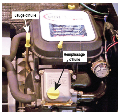
Schéma 4.3 — Jauge et remplissage d'huile, 12, 14, 16, 17 et 20 kW
