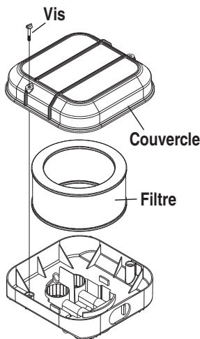
Schéma 4.5 — Filtre à air du moteur de 13, 14, 16, 17 et 20 kW
