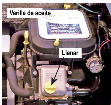
Figura 4.3 — Varilla de aceite y llenado, 12, 14, 16, 17 & 20kW
