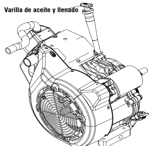
Figura 4.1 — Varilla de aceite y llenado, 8kW
