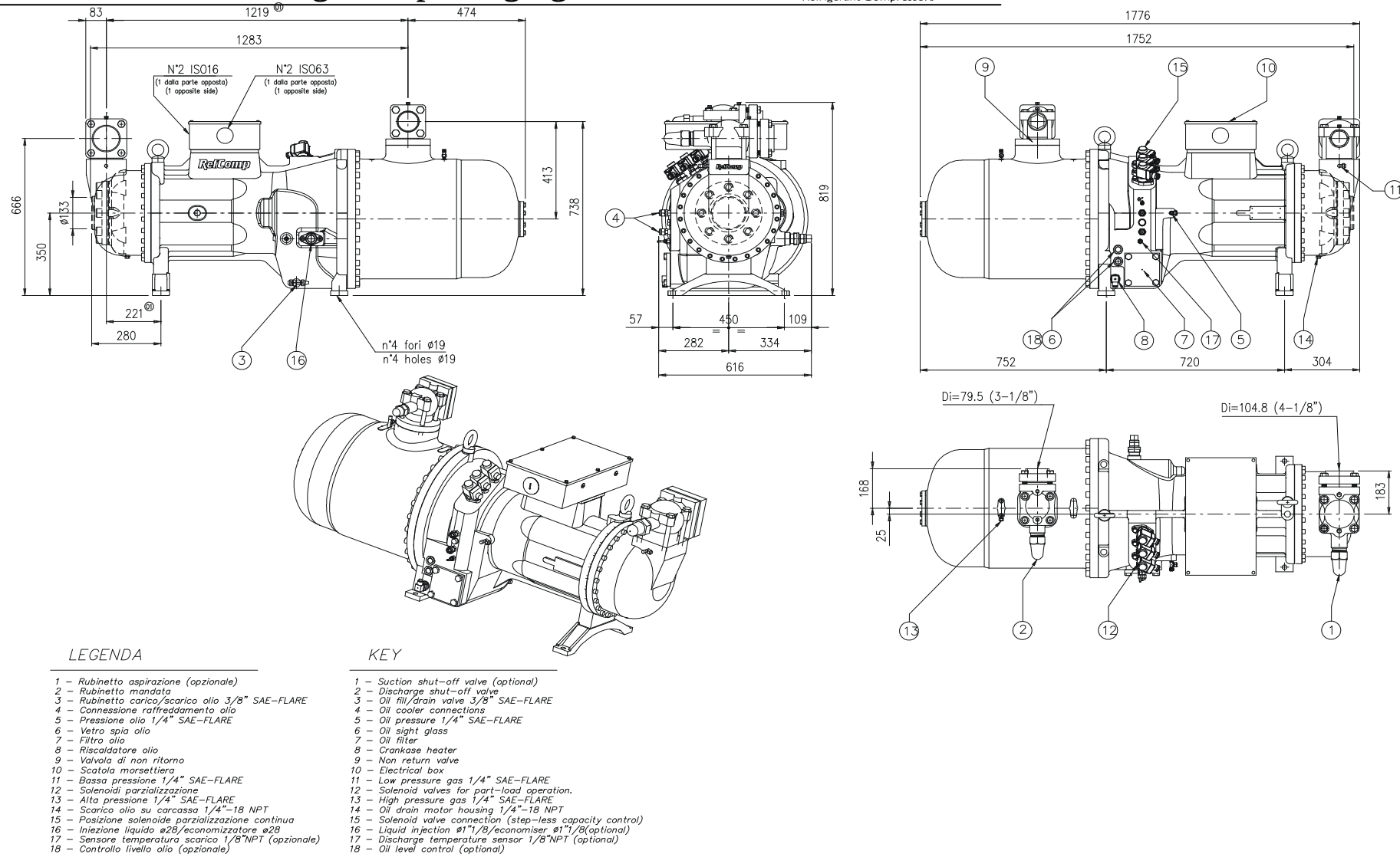
Figura 8-G: dimensioni SRC-S-755 (MSI080 r.00);
