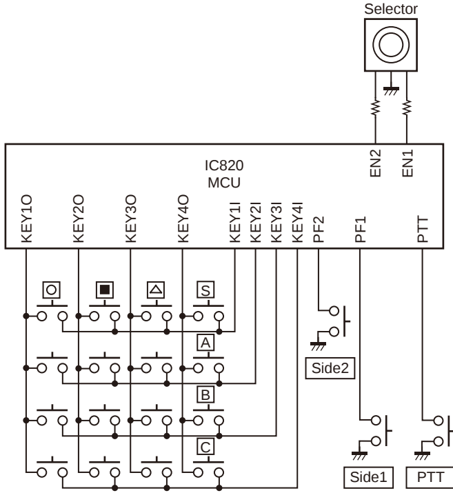
Fig. 10 Key input
