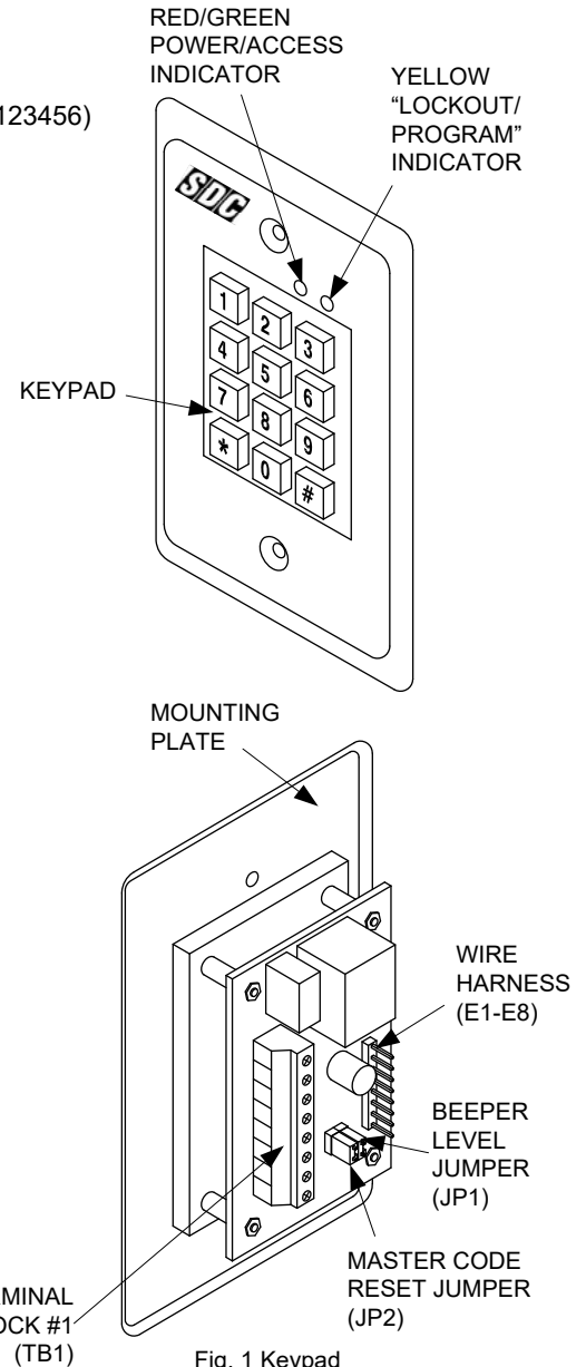
Fig. 1 Keypad
