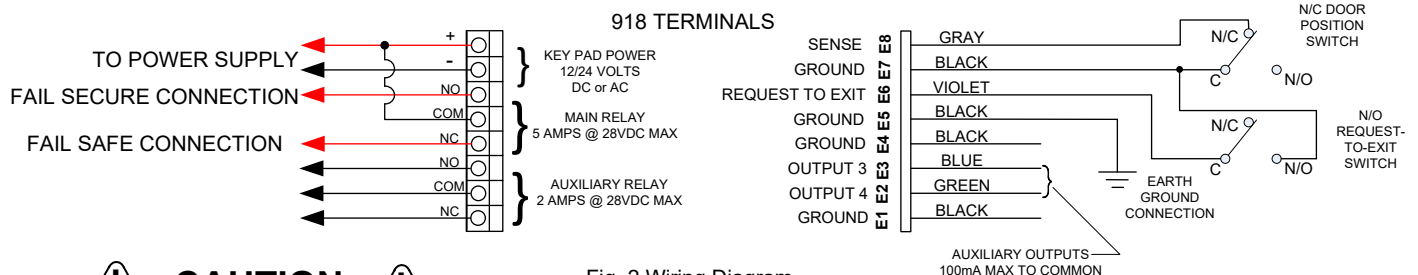
Fig. 2 Wiring Diagram
