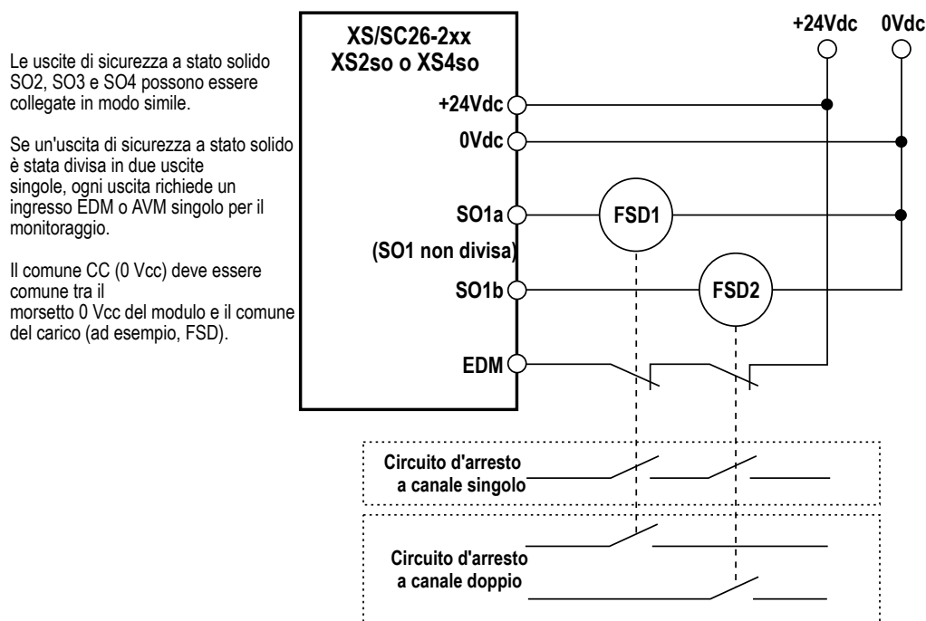
Figura 43. Collegamento XS/SC26-2 generico: Uscita di sicurezza a stato solido con EDM
