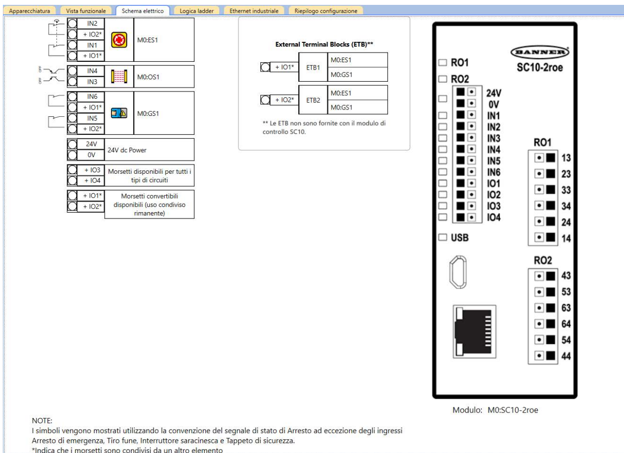
Figura 252. Scheda Schema elettrico con pulsante di arresto di emergenza, sensore ottico, interruttore saracinesca e morsettiere esterne
