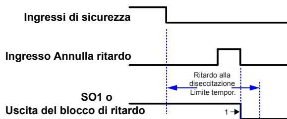
Figura 28. L'ingresso di sicurezza rimane in modalità arresto
