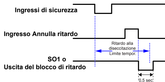
Figura 29. Funzione Diseccita uscita
