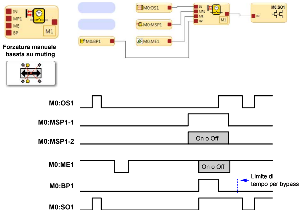
Figura 121. Forzatura manuale basata sul muting
