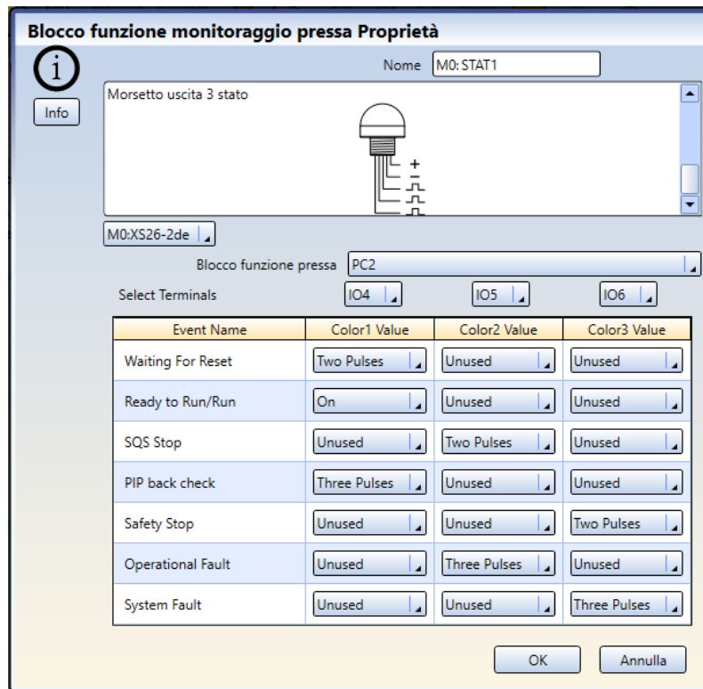
Figura 49. Monitoraggio proprietà del blocco funzione pressa
