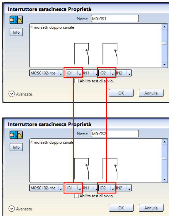
Figura 4. GS1 e GS2 condividono IO1 e IO2
