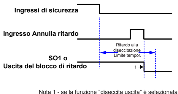
Figura 21. L'ingresso di sicurezza rimane in modalità arresto
