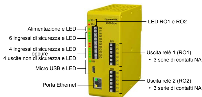
Figura 7. Caratteristiche e indicatori
