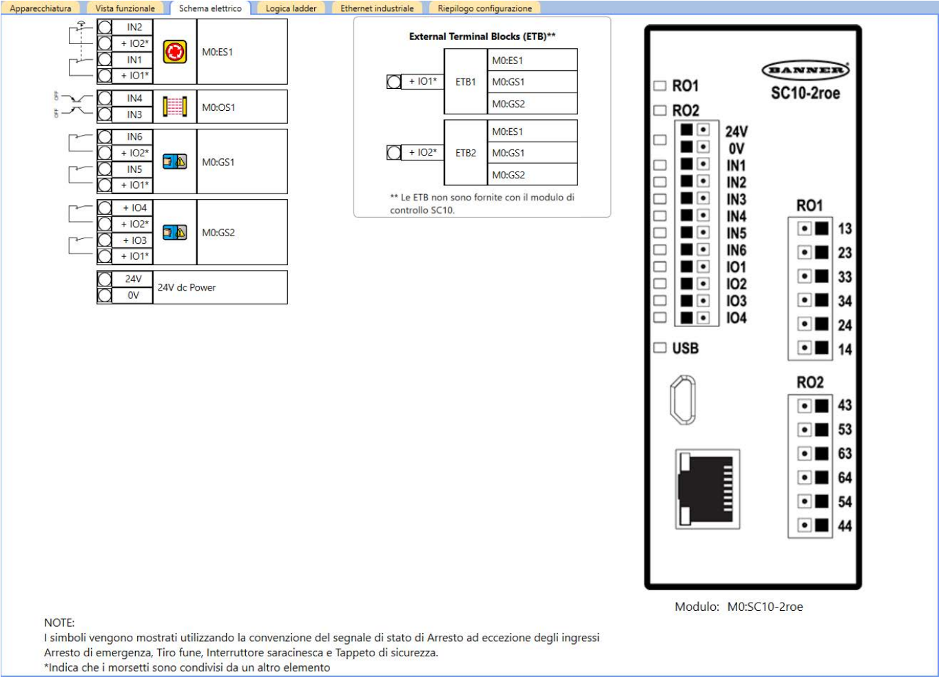
Figura 78. Scheda Schema elettrico : SC10-2 con morsettiere esterne
