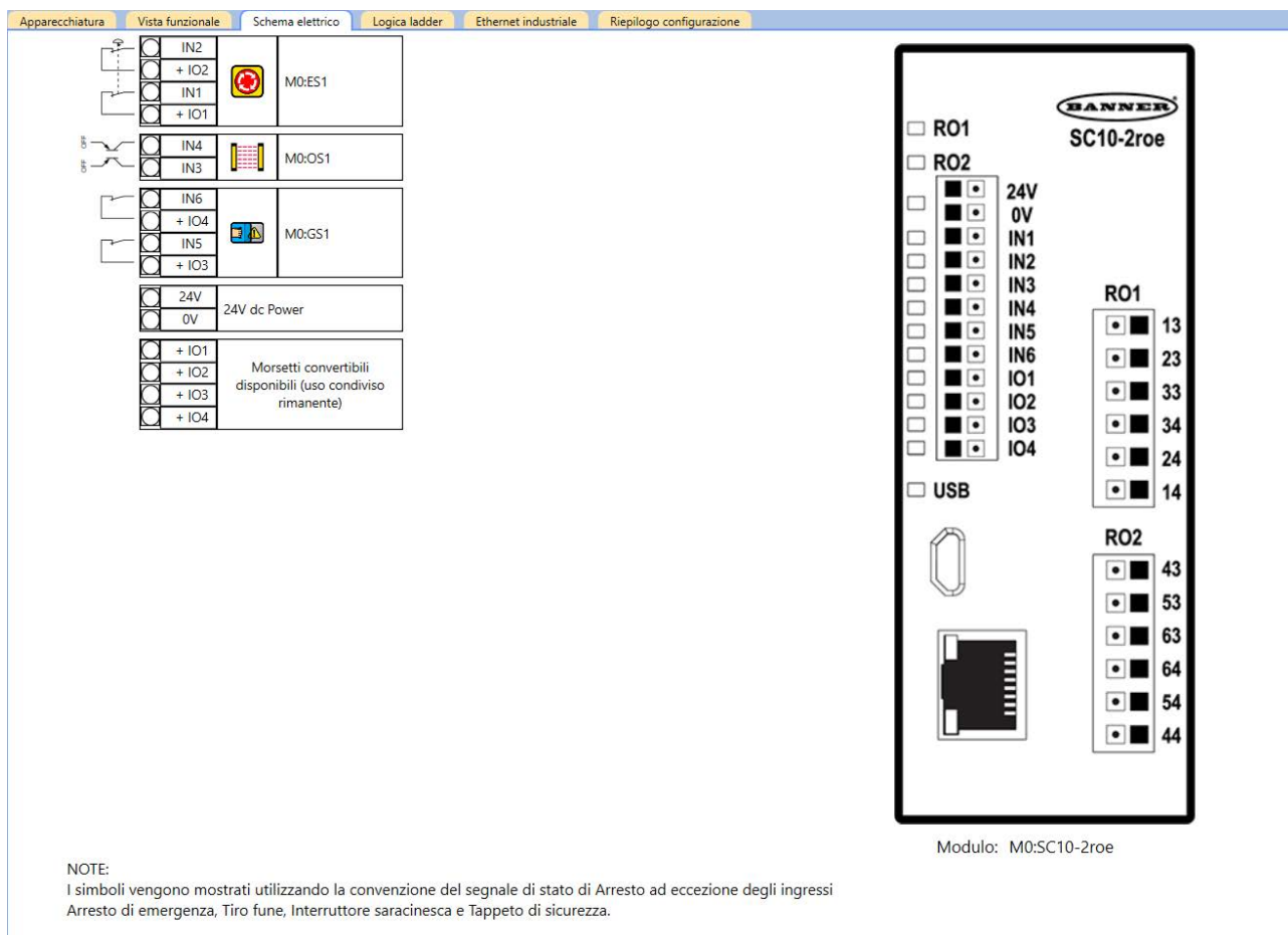
Figura 247. Scheda Schema elettrico con pulsante di arresto di emergenza, sensore ottico e interruttore saracinesca
