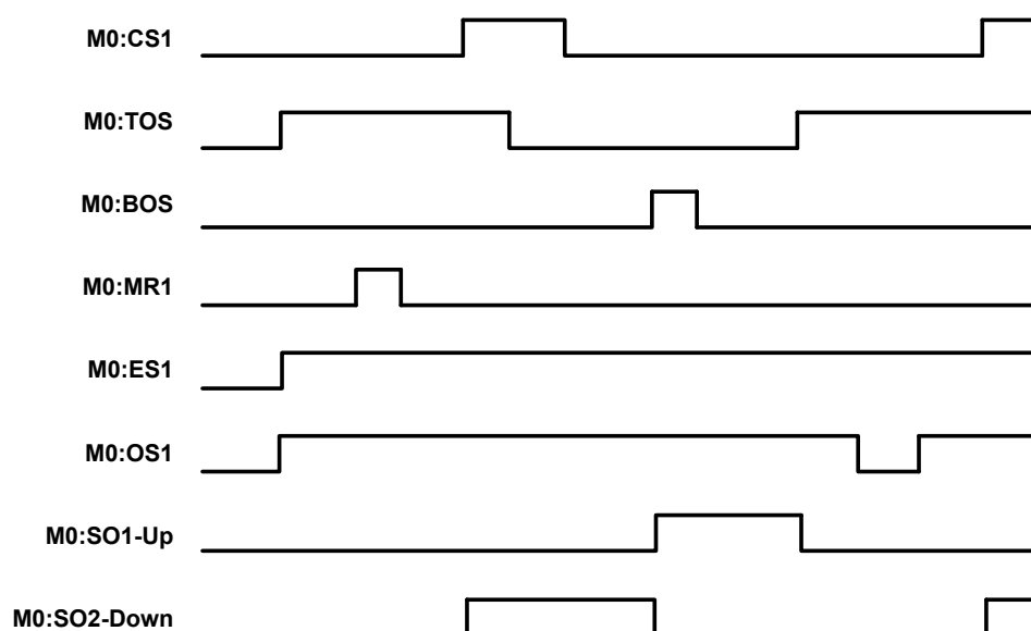
Figura 138. Diagramma dei tempi di controllo pressa, comando a singolo attuatore
