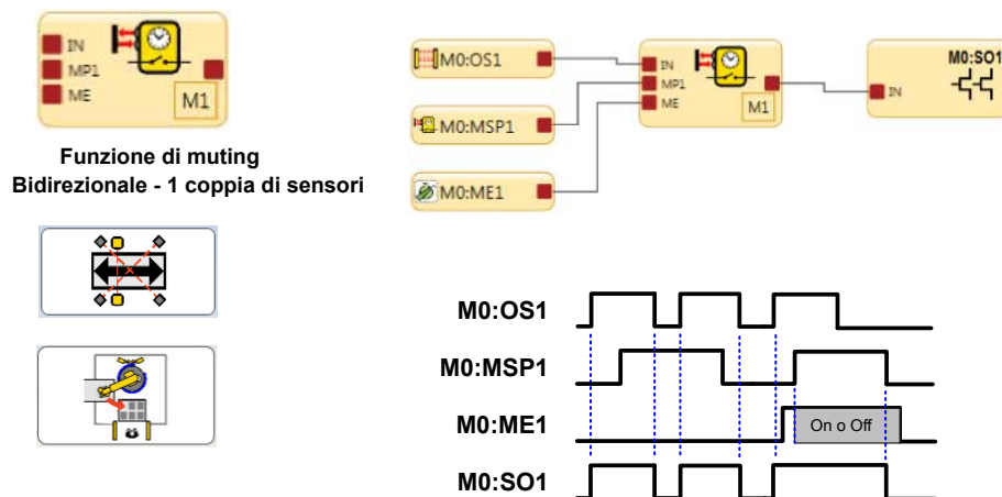
Figura 125. Diagramma dei tempi - Blocco di muting bidirezionale, una coppia di sensori con muting
