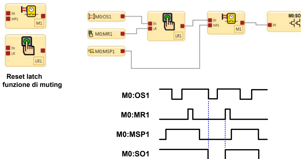
Figura 118. Diagramma dei tempi - Blocco reset latch e blocco di muting
