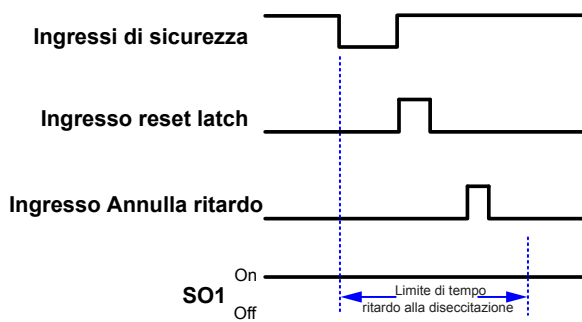
Figura 23. Funzione Tieni uscita eccitata per ingressi di sicurezza con reset di tipo latch
