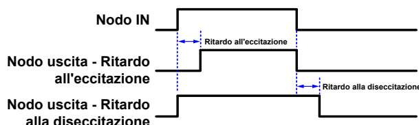
Figura 110. Diagramma dei tempi blocco di ritardo
