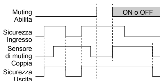
Figura 128. Logica di temporizzazione: una coppia di sensori con funzione di muting e Abilita muting
