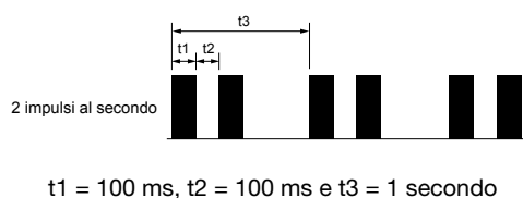
Figura 47. 2 impulsi al secondo
