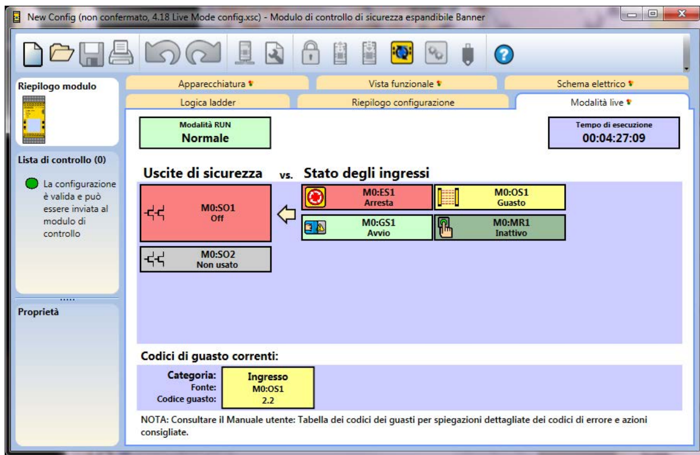
Figura 94. Tempo di esecuzione—Scheda Modalità live XS/SC26-2
