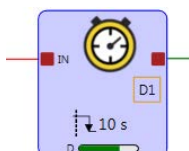
Figura 106. Ritardo uscita—Solo moduli di controllo di base XS/SC26-2 FID 2 o versioni successive e SC10-2
