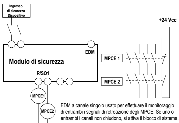
Figura 38. Collegamento EDM a un canale
