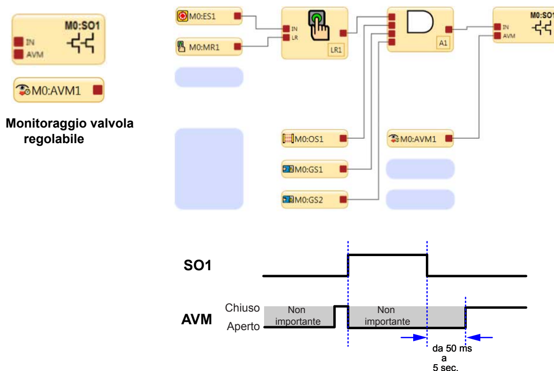
Figura 20. Logica di temporizzazione — Funzione AVM
