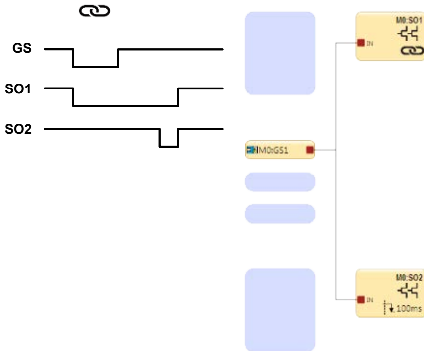
Figura 35. Diagramma dei tempi - uscite di sicurezza collegate
