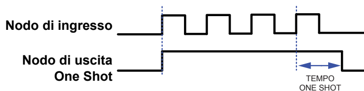
Figura 131. Diagramma dei tempi Heartbeat One Shot
