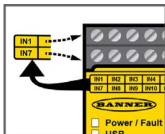
Figura 16. XS/SC26-2 – Posizioni dei morsetti di ingresso e uscita
