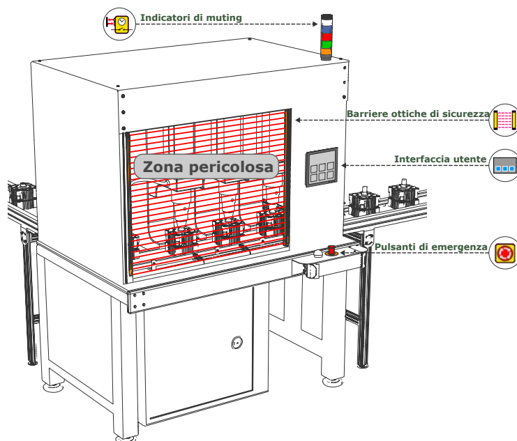
Figura 15. SC10-2 - Applicazione di esempio
