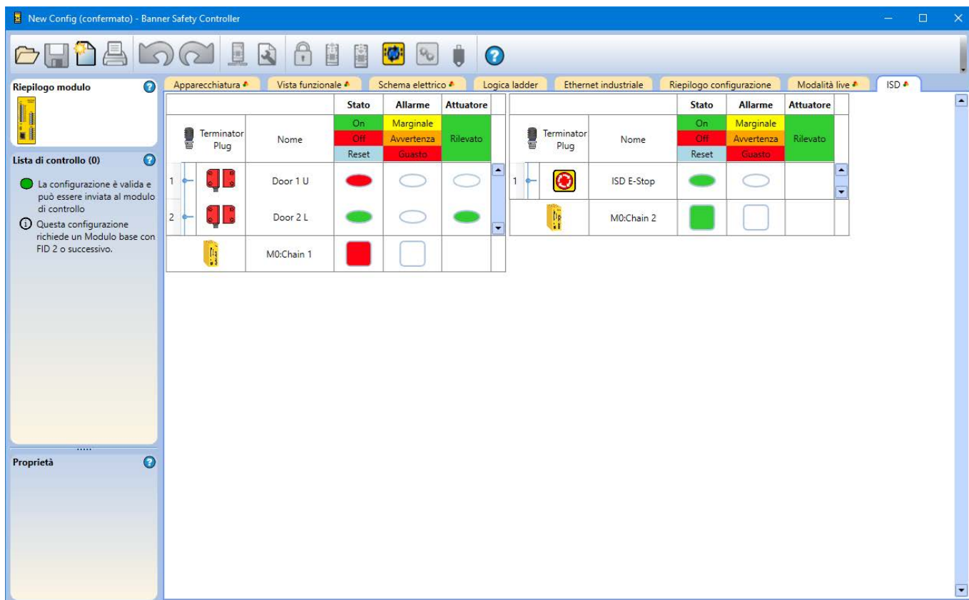
Figura 81. Scheda ISD in Modalità live con un interruttore aperto
