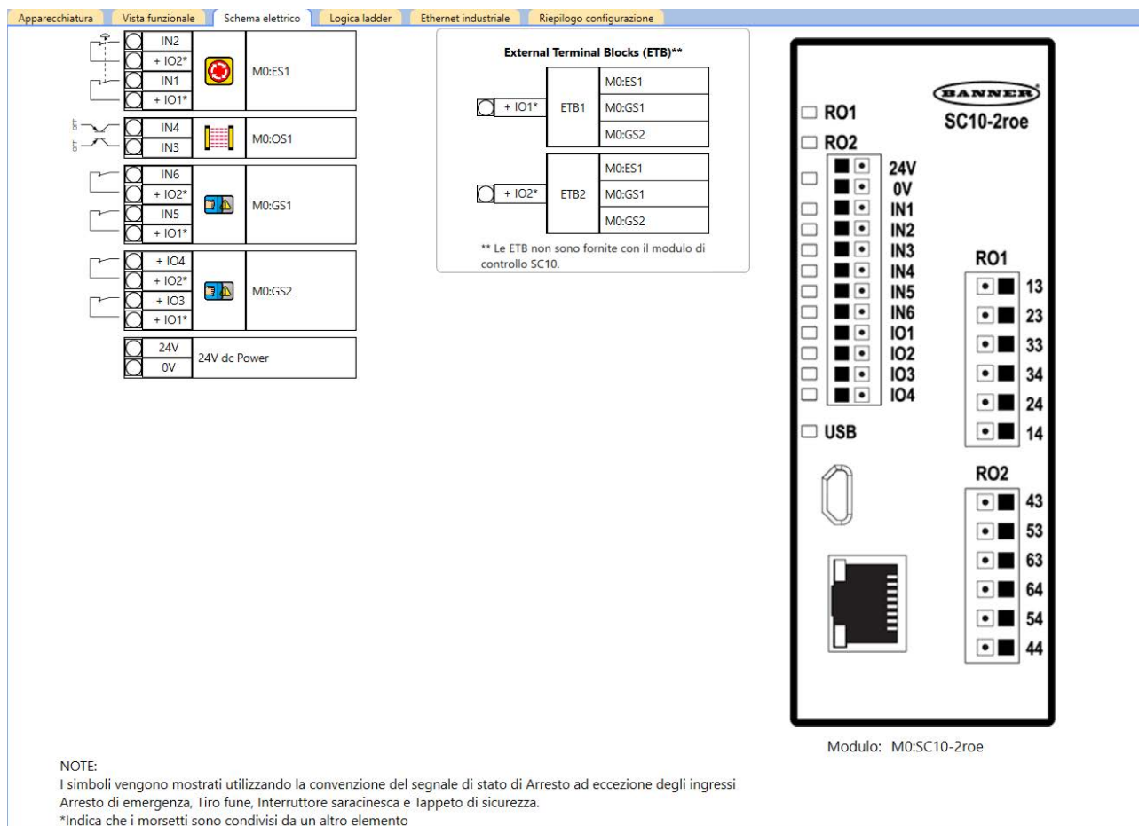
Figura 248. Scheda Schema elettrico con tre pulsanti di emergenza e morsettiere esterne
