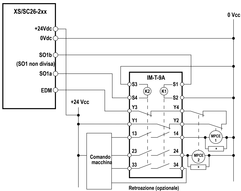
Figura 45. Collegamento XS/SC26-2 generico: Uscita di sicurezza a stato solido per IM-T-9A
