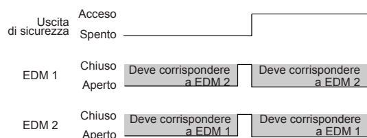
Figura 42. Logica di temporizzazione: Stato EDM a due canali, rispetto all'uscita di sicurezza
