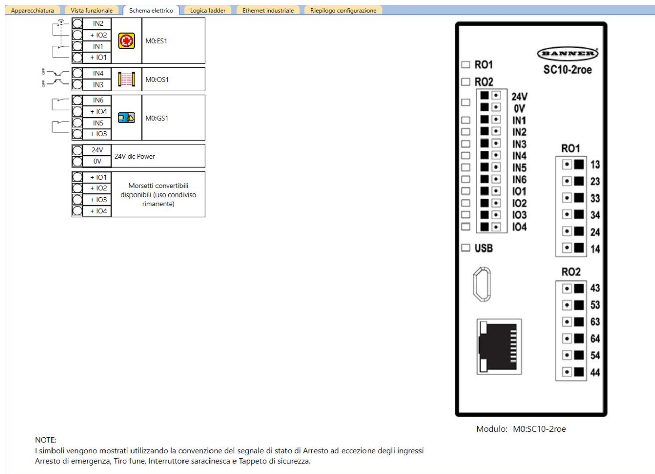
Figura 250. Scheda Schema elettrico con pulsante di arresto di emergenza, sensore ottico e interruttore saracinesca
