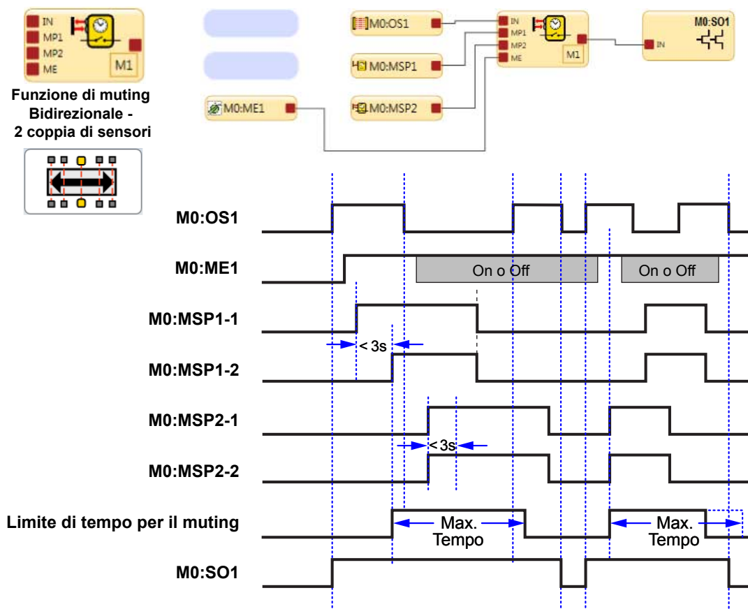
Figura 127. Arresto di emergenza e funzione muting
