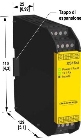
Figura 12. Dimensioni del modulo di espansione
