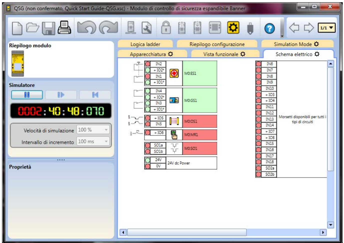
Figura 101. Modalità simulazione - scheda Schema elettrico
