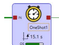
Figura 107. Solo blocco One Shot—XS/SC26-2 FID 4 o moduli di controllo di base versioni successive
