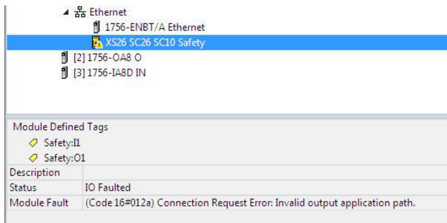
Figura 166. Errato: VRCD più ISD su un modulo di controllo di sicurezza che non supporta questa funzione
