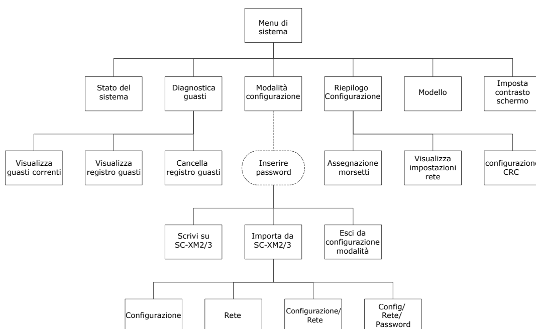
Figura 148. Schema dell'interfaccia integrata
