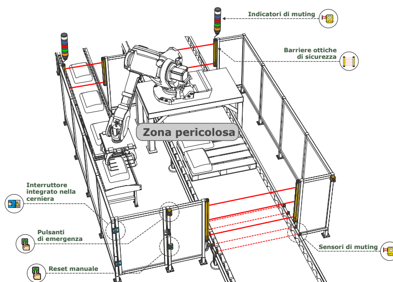
Figura 14. Applicazioni di esempio - cella robotica
