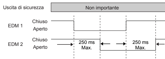
Figura 41. Logica di temporizzazione: EDM a due canali, sincronizzazione tra canali
