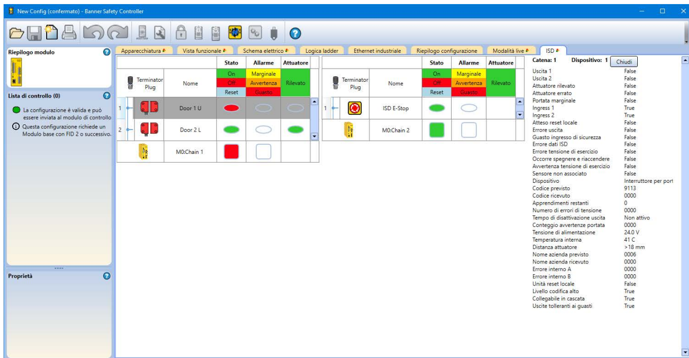
Figura 82. Scheda ISD in Modalità live con dati diagnostici
