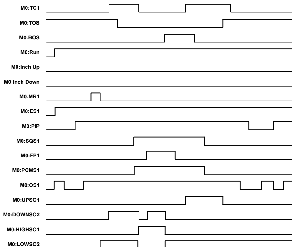
Figura 140. Diagramma dei tempi di controllo pressa con impostazione della corsa ascendente manuale
