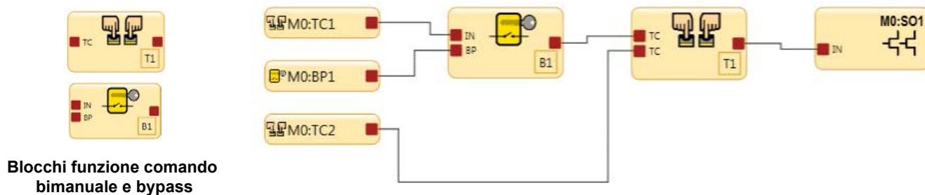
Figura 145. Diagramma dei tempi — Blocco comando bimanuale e blocchi di bypass con 2 ingressi comando bimanuale
