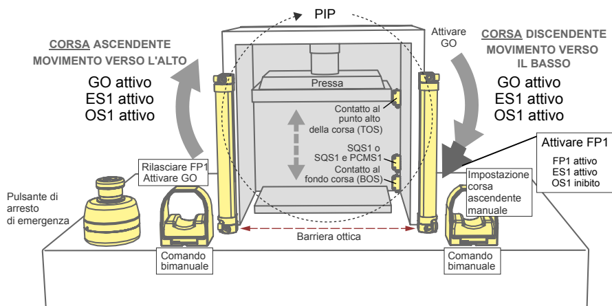
Figura 64. Configurazione di esempio del controllo pressa con tutte le funzionalità
