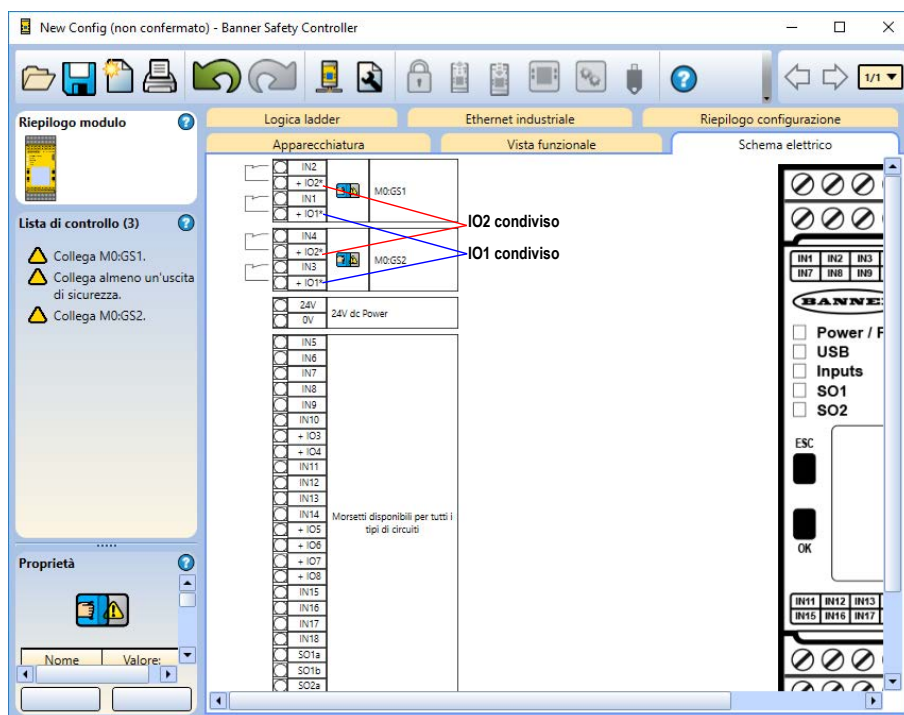
Figura 5. Vista della scheda Schema elettrico con gli I/O condivisi
