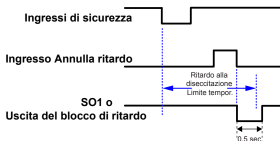
Figura 22. Funzione Diseccita uscita
