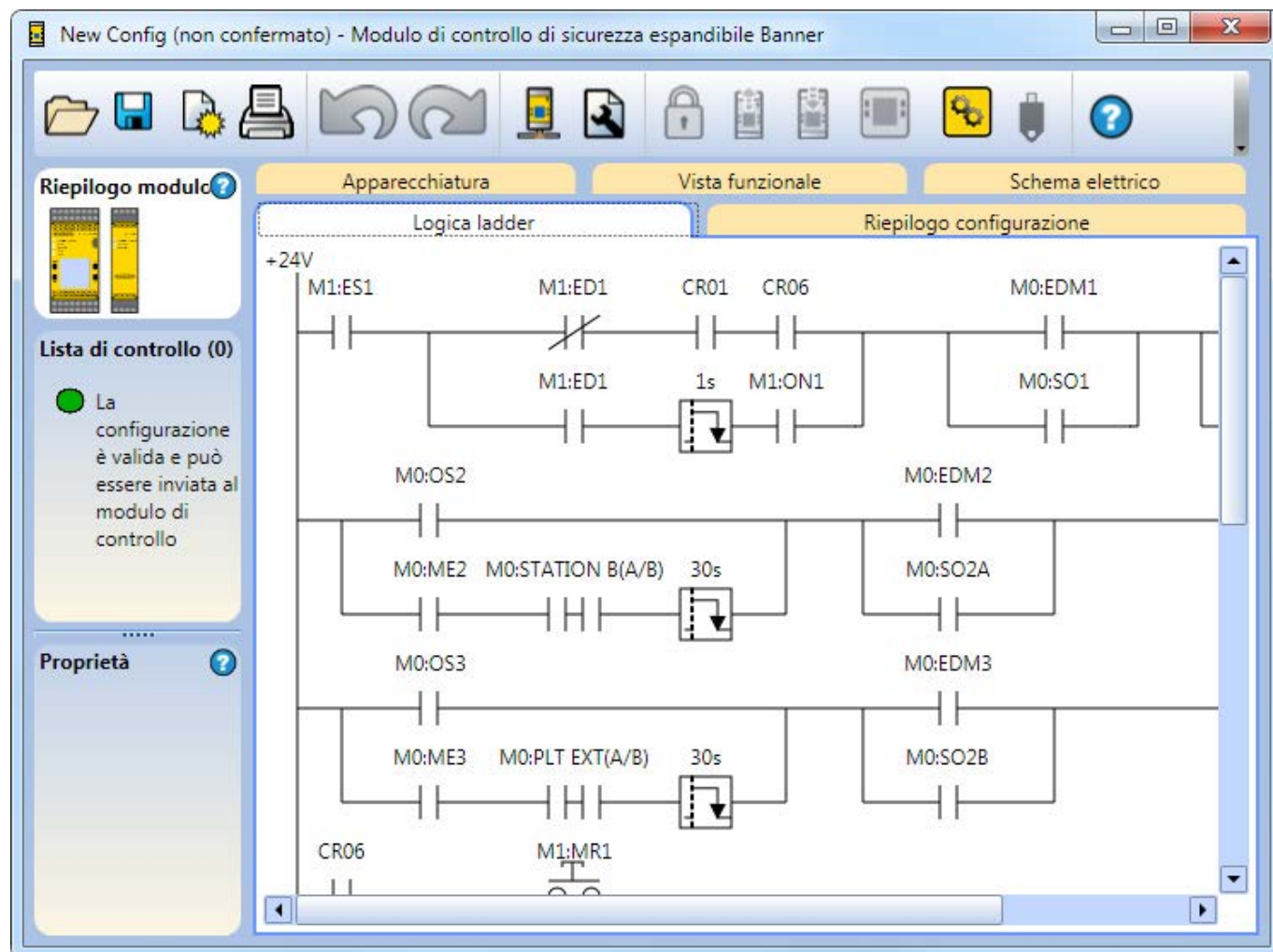
Figura 79. Scheda Logica ladder
