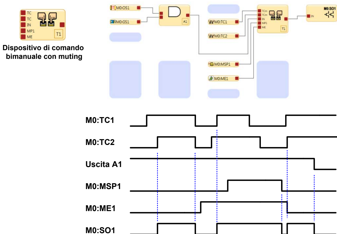
Figura 147. Diagramma dei tempi - Blocco comando bimanuale con muting
