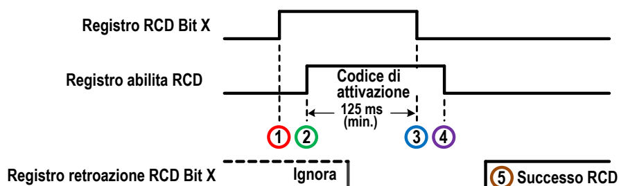
Figura 27. Sequenza di reset virtuale o Annulla ritardo (RCD) - Metodo temporizzato
