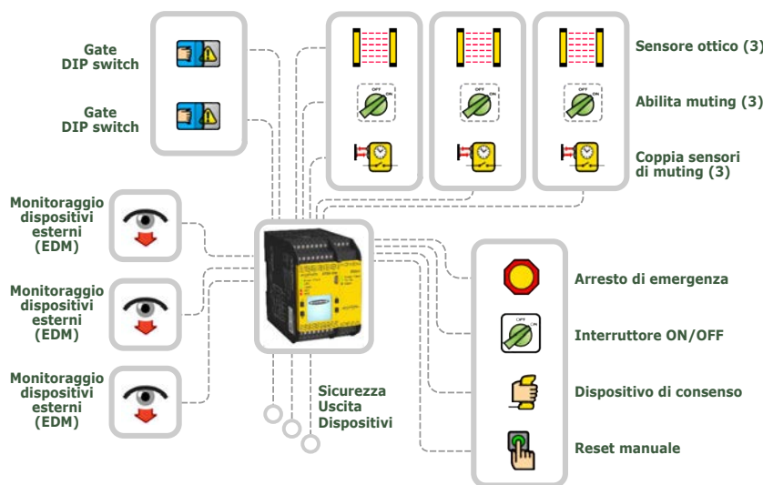
Figura 58. Schema della configurazione di esempio
