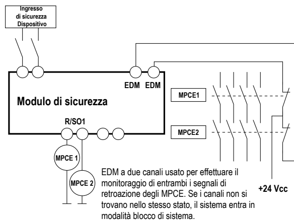
Figura 39. Collegamento EDM a due canali
