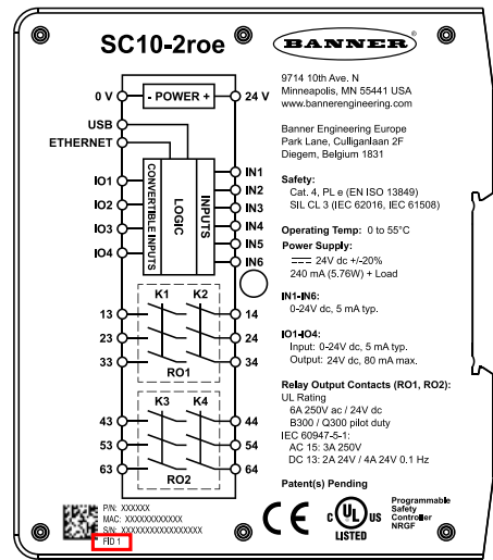
Figura 8. Esempio di etichetta SC10-2
