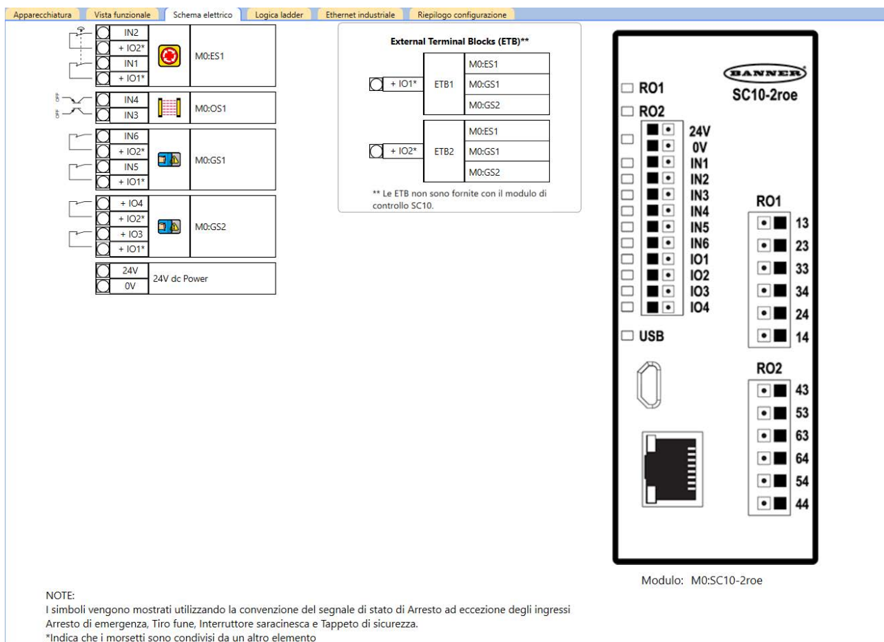
Figura 253. Scheda Schema elettrico con pulsante di arresto di emergenza, sensore ottico, interruttori saracinesca e morsettiere esterne
