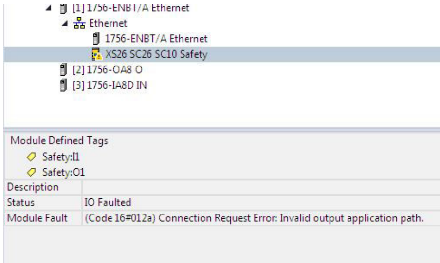
Figura 164. Errato: uso di segnali di stato/guasto ingresso virtuale in un modulo di controllo di sicurezza che non supporta questa funzione
