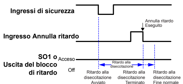
Figura 31. Funzione Tieni uscita eccitata per ingressi di sicurezza senza reset di tipo latch
