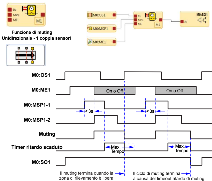
Figura 123. Diagramma dei tempi - Blocco di muting unidirezionale, una coppia di sensori con muting
