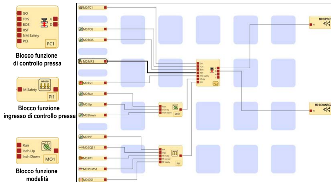
Figura 139. Configurazione di esempio per controllo pressa
