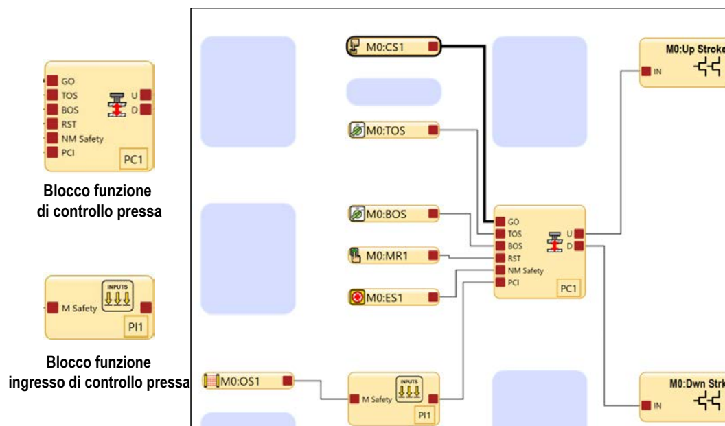
Figura 137. Esempio di configurazione per una piccola pressa
