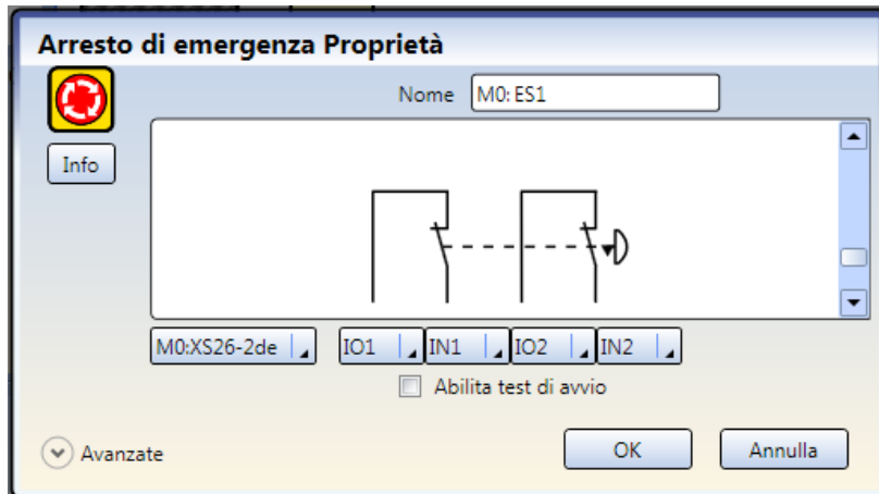
Figura 53. Impostazioni di base dell'ingresso di sicurezza
