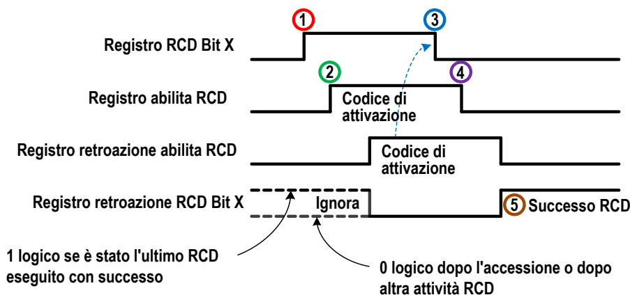
Figura 26. Sequenza di reset virtuale o Annulla ritardo (RCD) - Metodo segnale di retroazione
