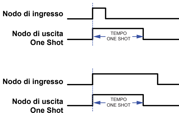
Figura 130. Diagrammi tipici dei tempi One Shot normali
