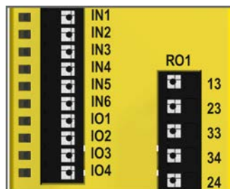
Figura 17. SC10-2 - Posizioni dei morsetti di ingresso e uscita
