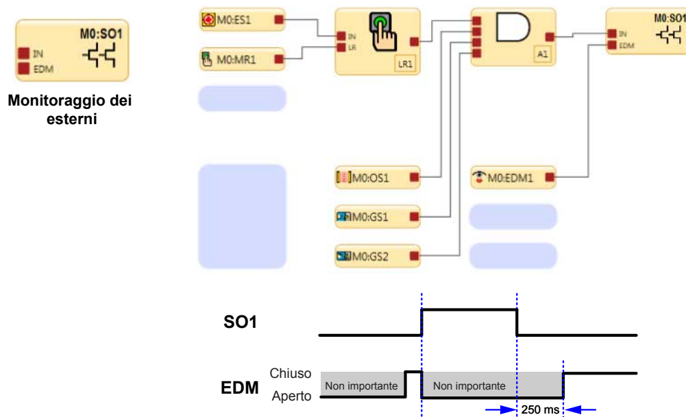
Figura 40. Logica di temporizzazione: Stato EDM a un canale, rispetto all'uscita di sicurezza
