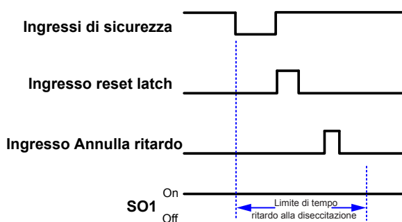
Figura 30. Funzione Tieni uscita eccitata per ingressi di sicurezza con reset di tipo latch
