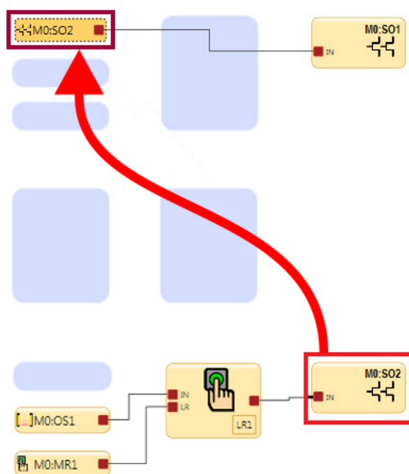
Figura 108. Uscita di sicurezza controllata da un'altra uscita di sicurezza
