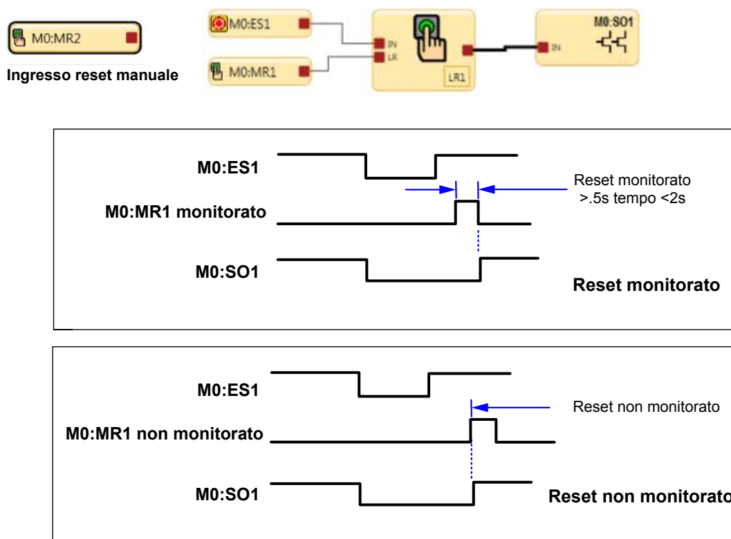
Figura 115. Diagramma dei tempi — Blocco reset latch, reset monitorato/non monitorato
