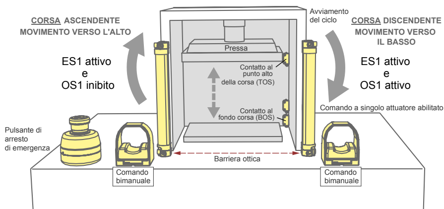
Figura 60. Esempio di configurazione semplice di controllo pressa
