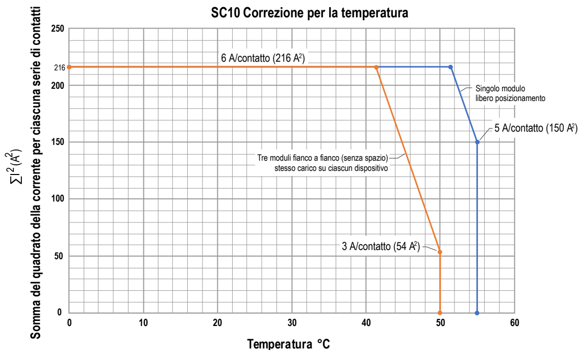
Figura 10. SC10-2 - Correzione per la temperatura
