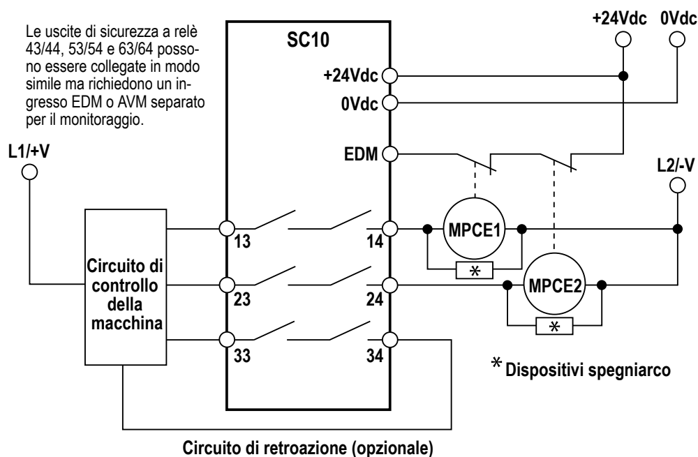
Figura 46. Collegamento SC10-2 generico: Uscita relè di sicurezza (doppio canale) con EDM
