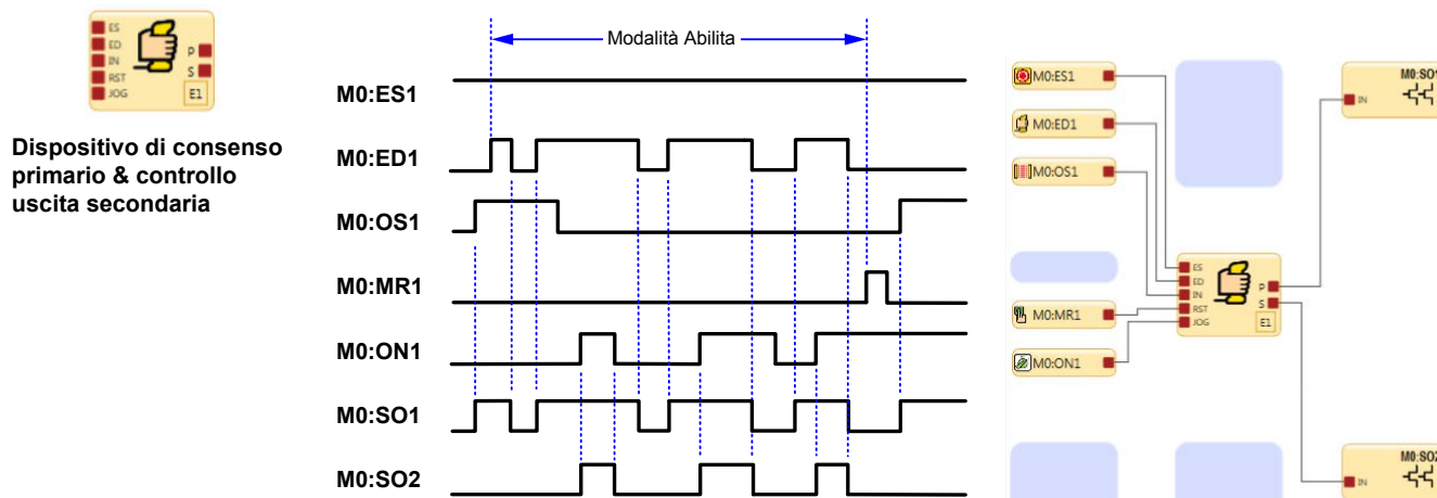
Figura 113. Diagramma dei tempi - dispositivo di consenso
