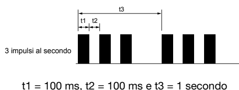
Figura 48. 3 impulsi al secondo
