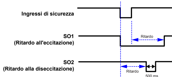
Figura 32. Diagramma dei tempi - ritardo all'eccitazione (On delay) e alla diseccitazione (Off delay) per uscita di sicurezza generica
