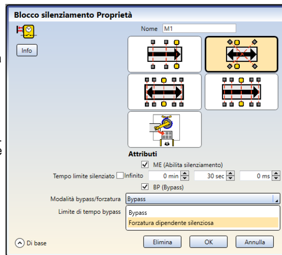
Figura 121. Forzatura manuale basata sul muting
