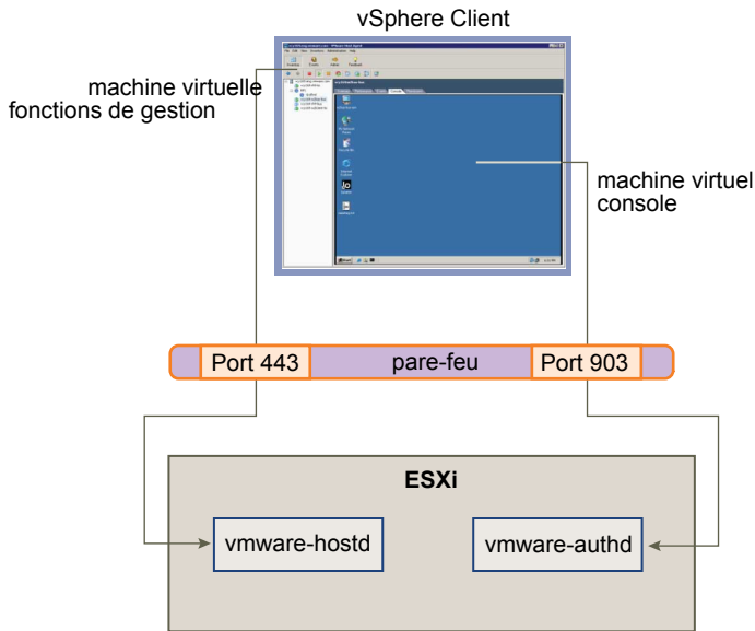
Figure 12-3. Utilisation des ports pour les communications client avec ESXi
