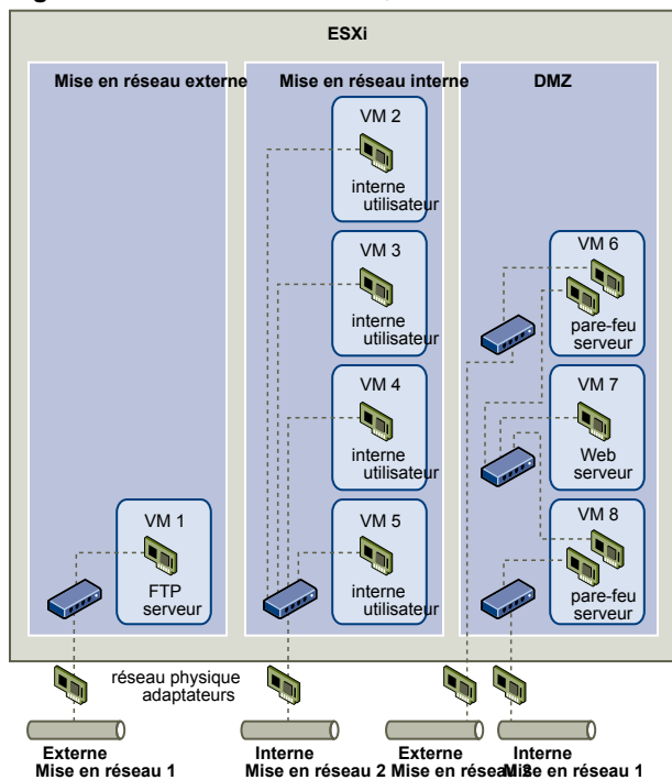
Figure 11-5. Réseaux externes, réseaux internes et DMZ configurée sur un hôte ESXi unique
