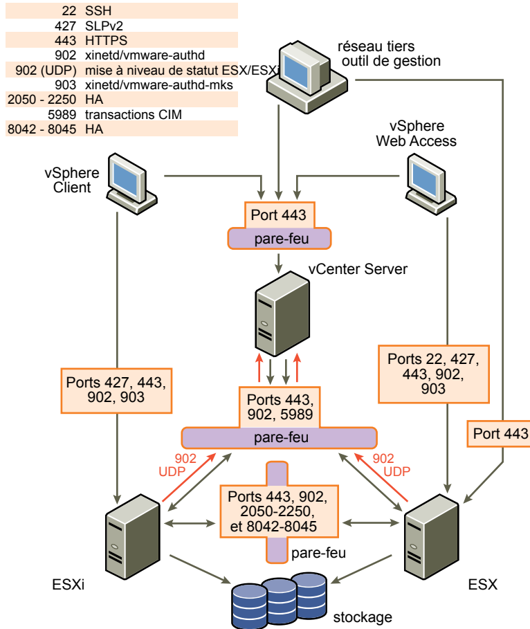
Figure 12-1. Exemple de configuration réseau vSphere et flux de trafic
