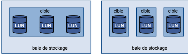
Figure 7-1. Représentations LUN et de cibles
