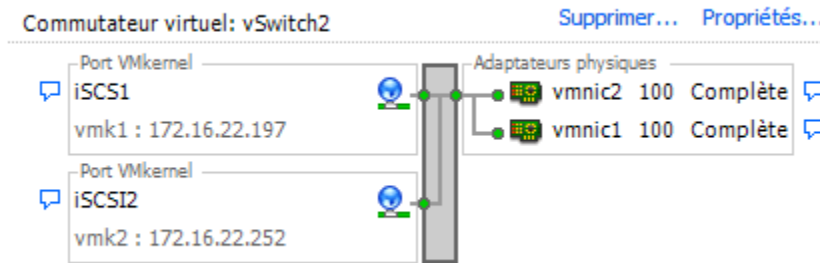
Figure 6-3. Ports iSCSI et NIC sur vSwitch unique
