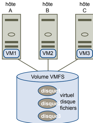
Figure 7-2. Partager un volume VMFS par le biais d'hôtes
