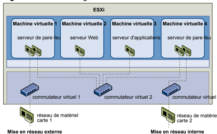
Figure 11-4. DMZ configurée sur un hôte ESXi
