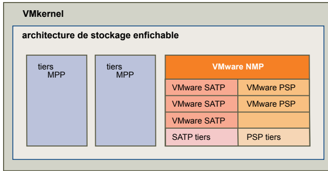
Figure 9-1. Architecture de stockage enfichable
