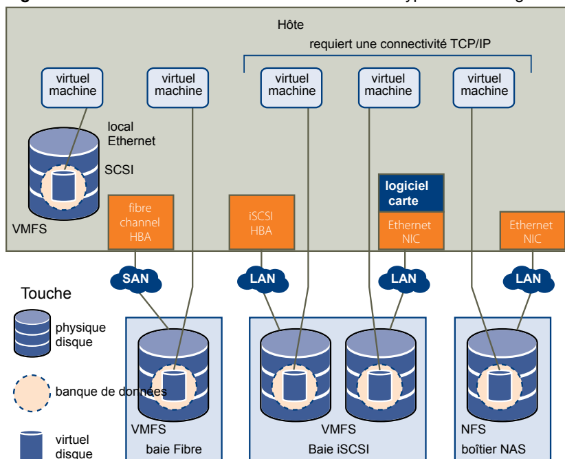
Figure 7-3. Machines virtuelles accédant à différents types de stockage
