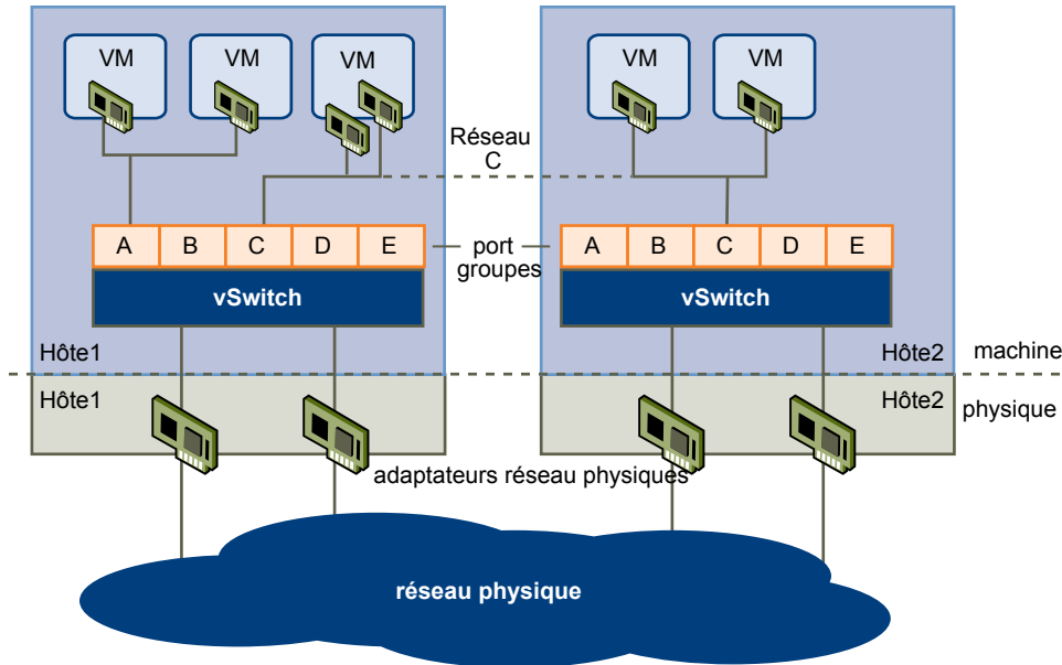
Figure 3-1. Réseau de commutateurs standard vNetwork
