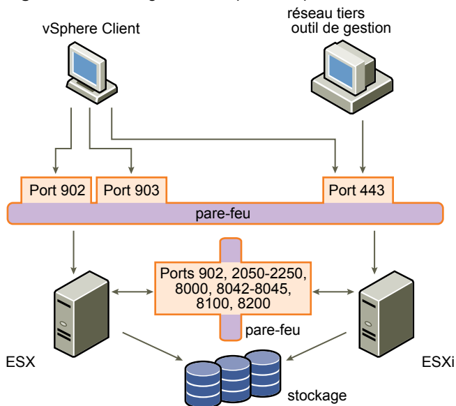
Figure 12-2. Configuration du pare-feu pour les réseaux ESXi gérés directement par un client
