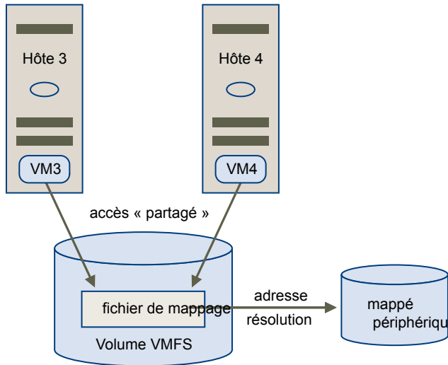
Figure 10-3. Accès à partir des machines virtuelles en clusters
