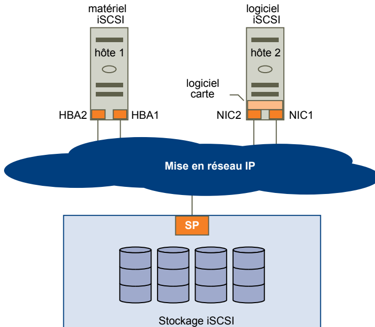
Figure 9-3. Chemins multiples basés sur l'hôte
