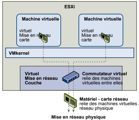
Figure 11-3. Mise en réseau virtuelle via l'utilisation de commutateurs virtuels
