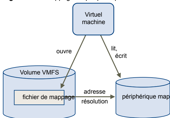
Figure 10-1. Mappage de périphérique brut
