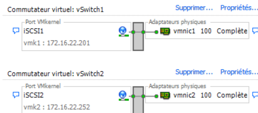
Figure 6-2. Ports iSCSI et NIC sur vSwitch distincts
