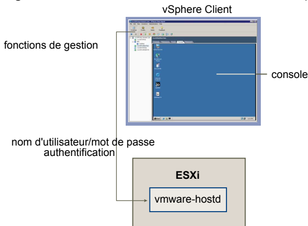
Figure 13-1. Authentification des communications du vSphere Client avec ESXi
