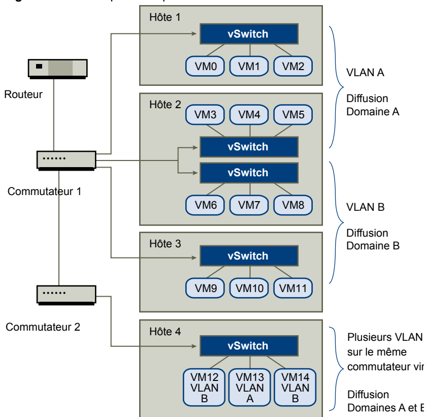
Figure 12-4. Exemple de disposition de VLAN
