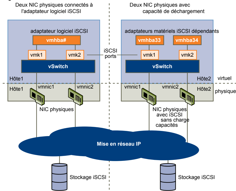
Figure 6-1. Mise en réseau avec iSCSI
