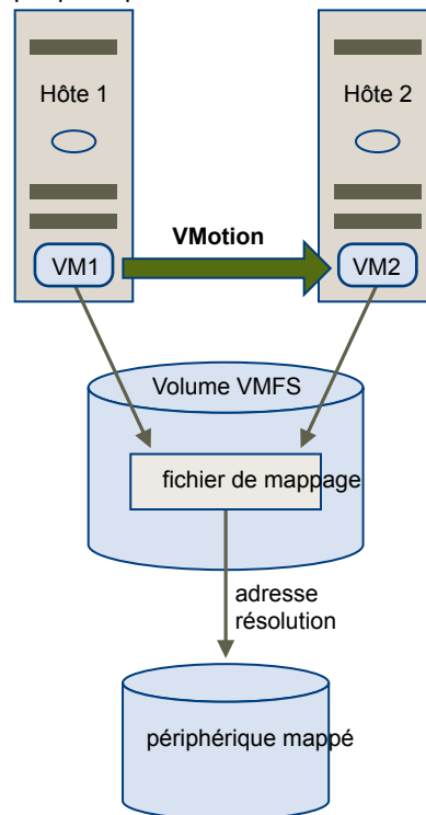
Figure 10-2. vMotion pour une machine virtuelle utilisant le mappage de périphérique brut
