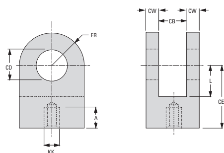
Plain Rod Clevis
