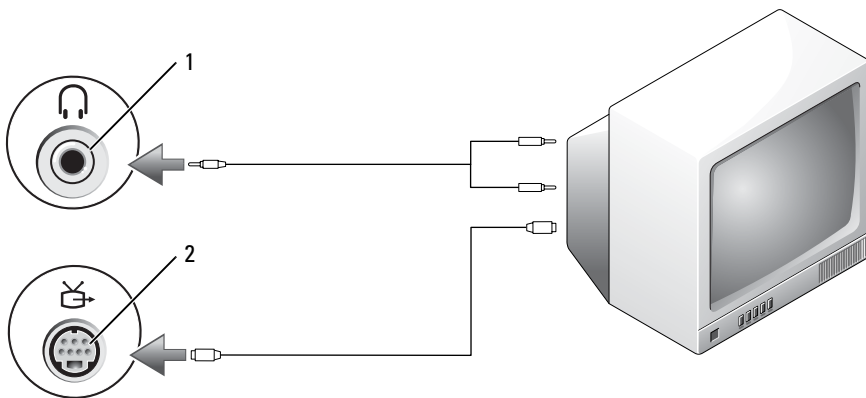
1 conector de áudio 2 conector de saída para TV S-video
