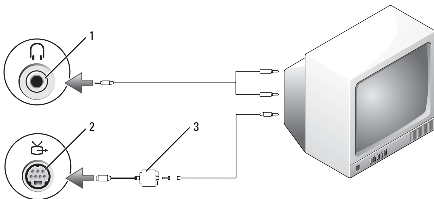
1 conector de entrada de áudio 2 conector de saída para TV S-vídeo 3 adaptador de vídeo composto
