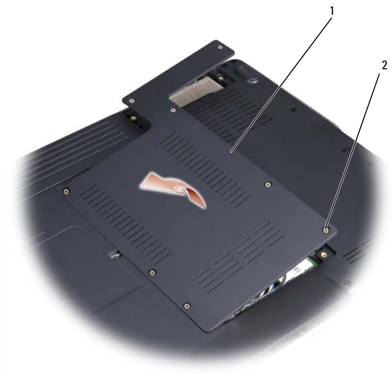
1 tampa 2 parafusos prisioneiros (5)
