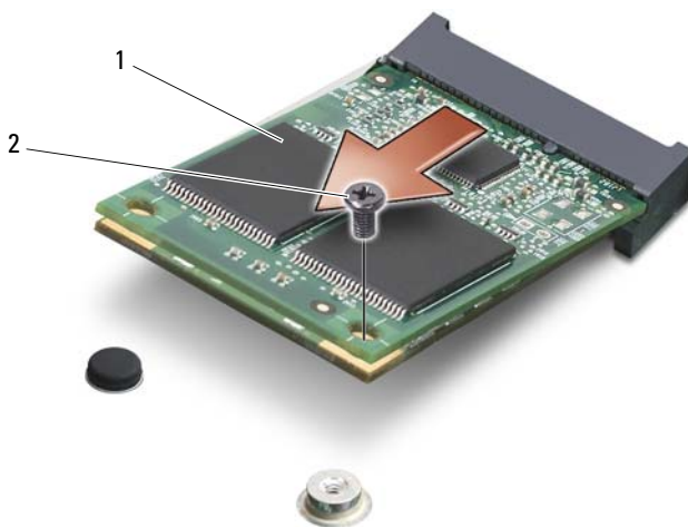
1 placa FCM 2 parafuso de fixação M2 x 3 mm
