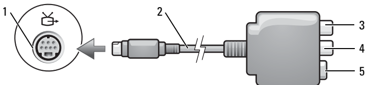
1 conector de saída para TV S-vídeo 2 adaptador de vídeo composto 3 conector de áudio digital S/PDIF 4 conector de saída de vídeo composto 5 conector S-vídeo
